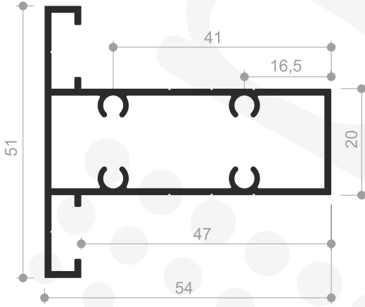
Profil No : 1006278 Ağırlık : 0,810 Kg/mt.
