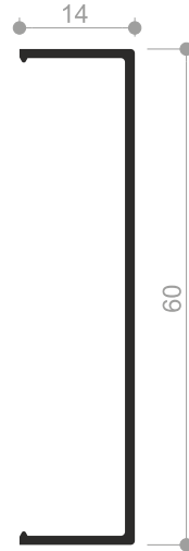
Profil No : 480690 Ağırlık : 0,290 Kg/mt.
