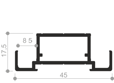
Profil No : 1006217 Ağırlık : 0,500 Kg/mt.
