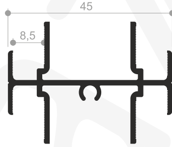
Profil No : 1006227 Ağırlık : 0,620 Kg/mt.
