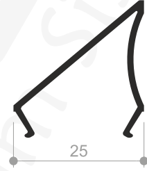
Profil No : 1006285 Ağırlık : 0,210 Kg/mt.
