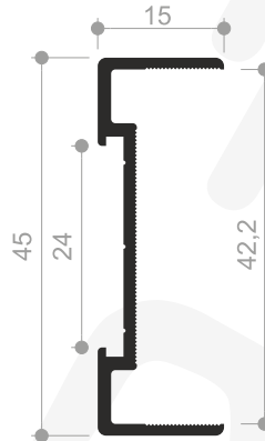
Profil No : 1506549 / Ağırlık : 0,330 Kg/mt.
