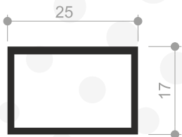
Profil No : 806 Ağırlık : 0,300 Kg/mt.
