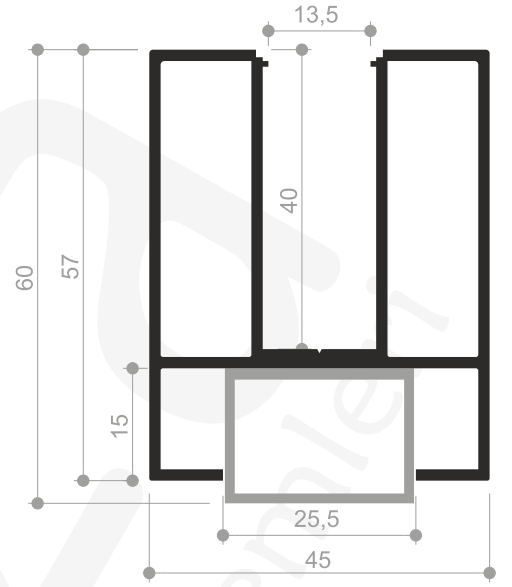
Profil No : 410648 Ağırlık : 1,200 Kg/mt.
