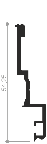
Profil No : 1506525 Ağırlık : 0,390 Kg/mt.
