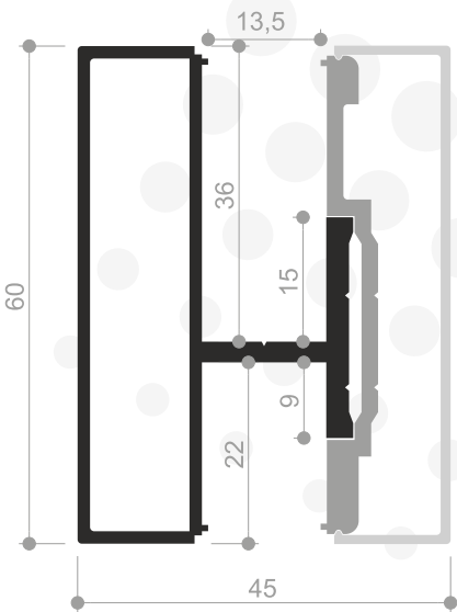
Profil No : 480692 Ağırlık : 0,900 Kg/mt.
