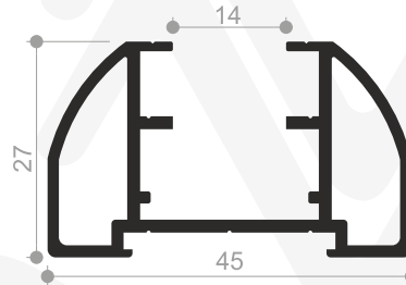
Profil No : 1506518 Ağırlık : 0,700 Kg/mt.
