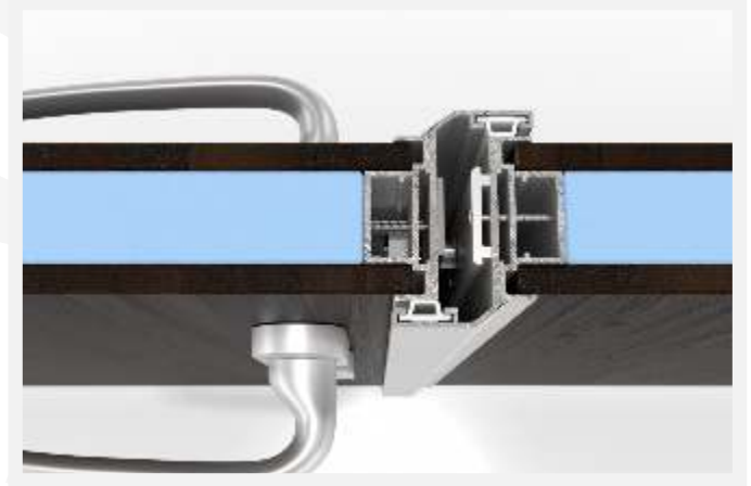
Açılır Çift Kanat (Çift Taraflı Sunta/MDF)
