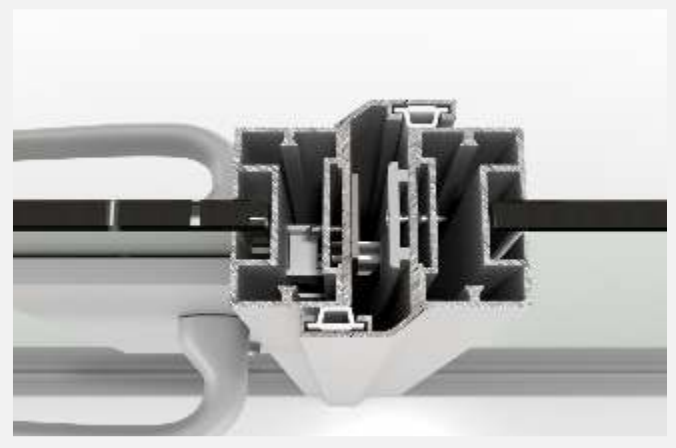
Açılır Çift Cam Kanat (Alüminyum Çerçevesi)
