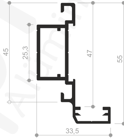
Profil No : 1406590 Ağırlık : 0,640 Kg/mt.
