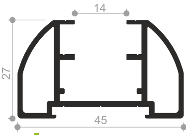
Profil No : 1506518 Ağırlık : 0,700 Kg/mt.
