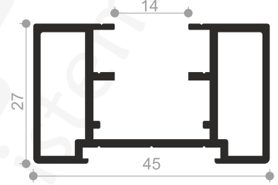
Profil No : 1506519 Ağırlık : 0,750 Kg/mt.
