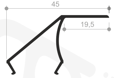
Profil No : 1006284 Ağırlık : 0,290 Kg/mt.
