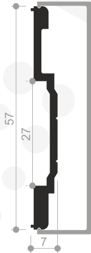
Profil No : 480691 Ağırlık : 0,425 Kg/mt.
