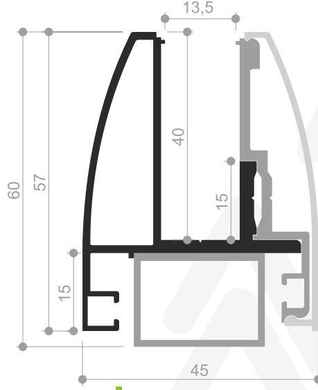
Profil No : 1006272 Ağırlık : 0,800 Kg/mt.
