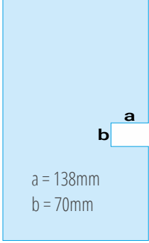
Çerçevesiz Cam Kanatlar İçin Kollu Yatay Kilit Düz Model
