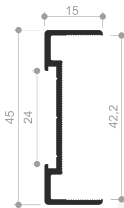
Profil No : 1506549 / Ağırlık : 0,330 Kg/mt.
