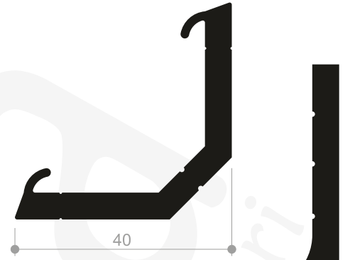
Profil No : 1406641 Ağırlık : 1,000 Kg/mt.
