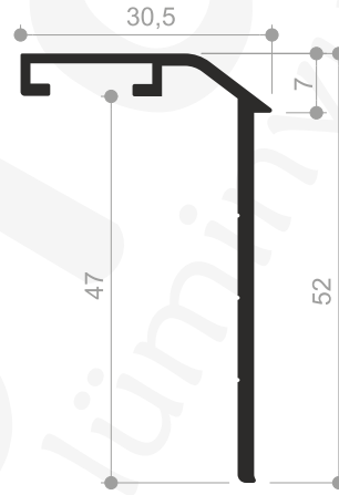
Profil No : 440682 Ağırlık : 0,420 Kg/mt.
