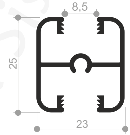
Profil No : 550630 Ağırlık : 0,370 Kg/mt.
