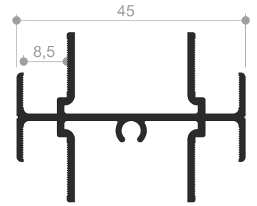
Profil No : 1006227 Ağırlık : 0,620 Kg/mt.
