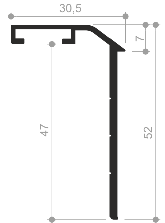
Profil No : 440682 Ağırlık : 0,420 Kg/mt.
