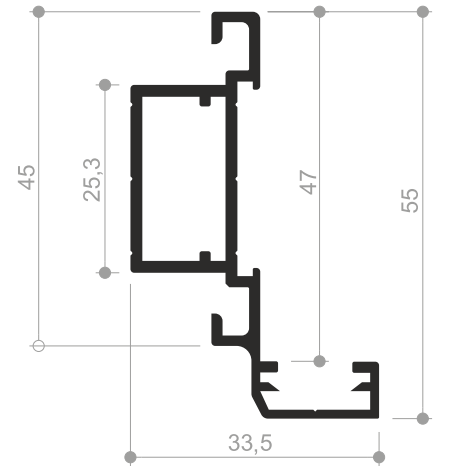
Profil No : 1406590 Ağırlık : 0,640 Kg/mt.
