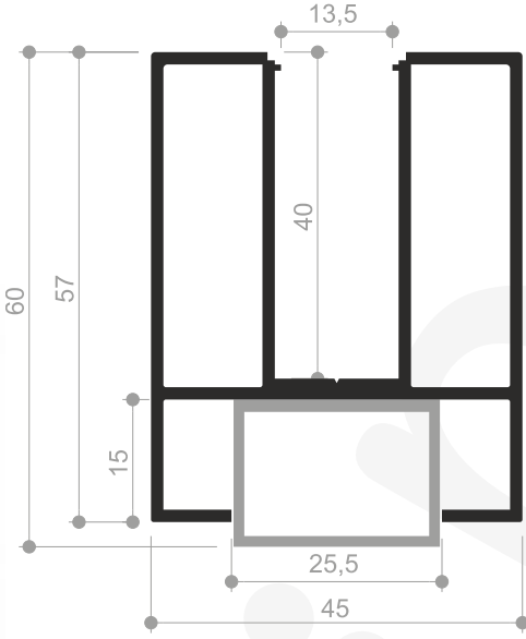
Profil No : 410648 Ağırlık : 1,200 Kg/mt.
