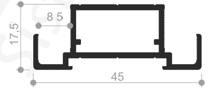
Profil No : 1006217 Ağırlık : 0,500 Kg/mt.
