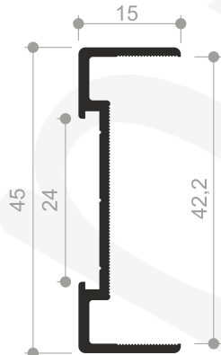
Profil No : 1506549 / Ağırlık : 0,330 Kg/mt.
