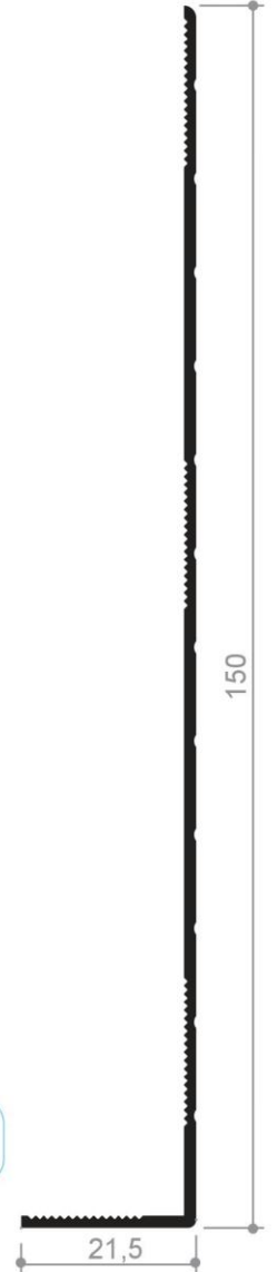
Profil No : 1006172 Ağırlık : 0,675 Kg/mt.
