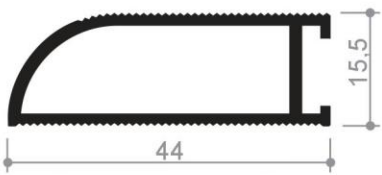
Profil No : 1006190 Ağırlık : 0,510 Kg/mt.
