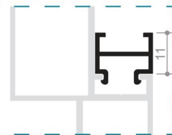
Profil No : 1406597 Ağırlık : 0,175 Kg/mt.
