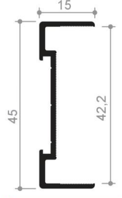
Profil No : 1506549 Ağırlık : 0,325 Kg/mt.
