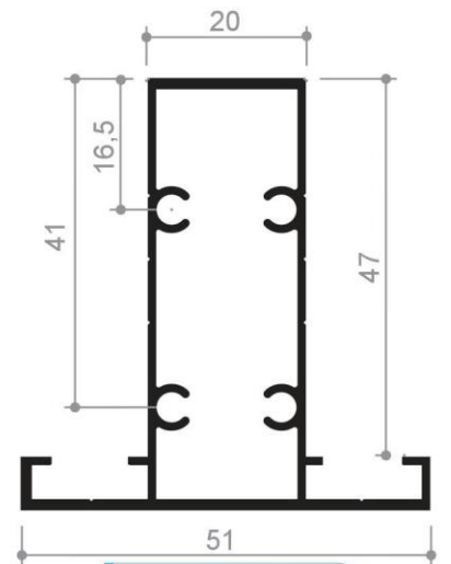
Profil No : 1006278 Ağırlık : 0,810 Kg/mt.
