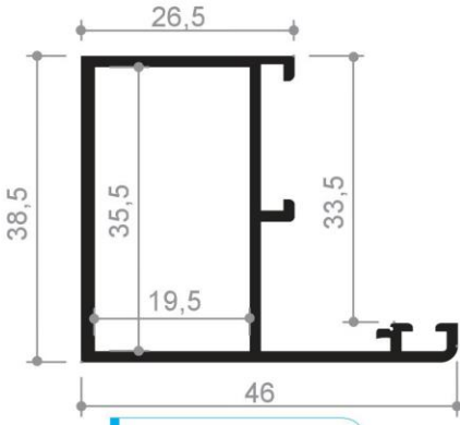
Profil No : 1506538 Ağırlık : 0,650 Kg/mt.
