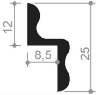
Profil No : 180695 Ağırlık : 0,250 Kg/mt.
