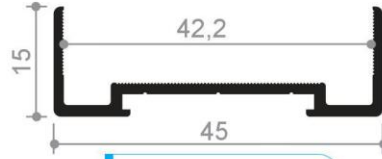
Profil No : 1506549 Ağırlık : 0,330 Kg/mt.
