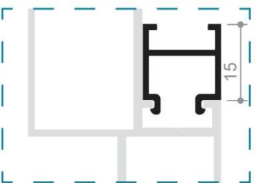
Profil No : 1006298 Ağırlık : 0,200 Kg/mt.
