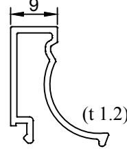
Profil No: 1006155 Ağırlık : 0.197 Kg/m
