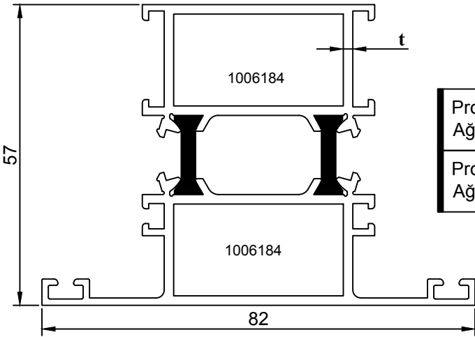
GENİŞ ORTA KAYIT PROFİLİ
