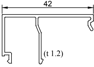
Profil No: 510677 Ağırlık : 0.305 Kg/m
