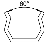
Profil No: 230665 Ağırlık : 0.238 Kg/m
