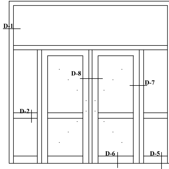
DIŞA AÇILAN KAPILARDA ADAPTÖR UYGULAMASI
