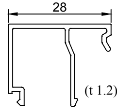
Profil No: 500651 Ağırlık : 0.262 Kg/m
