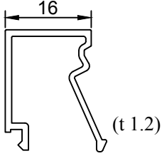
Profil No: 510686 Ağırlık : 0.208 Kg/m
