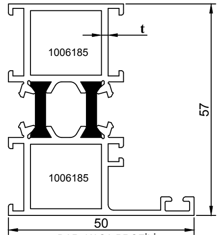
DAR KASA PROFİLİ
