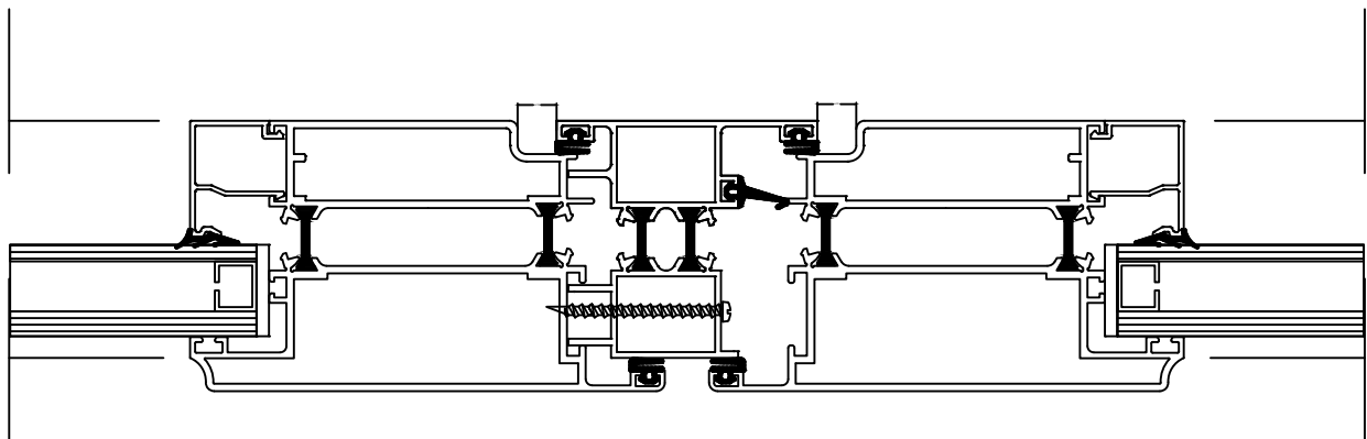
DETAY 8 DIŞA AÇILIR ÇİFT KAPI DETAYI
