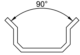
Profil No: 230664 Ağırlık : 0.254 Kg/m
