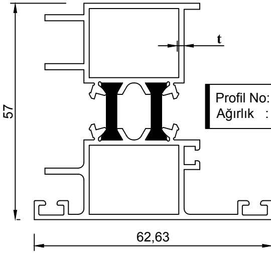
DIŞA AÇILIR KAPI PROFİLİ
