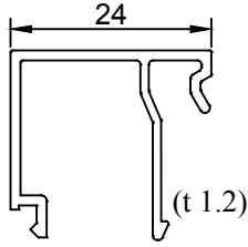
Profil No: 510675 Ağırlık : 0.246 Kg/m
