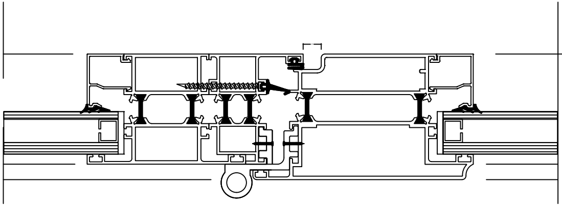
DETAY 7 DIŞA AÇILIR KAPI DETAYI
