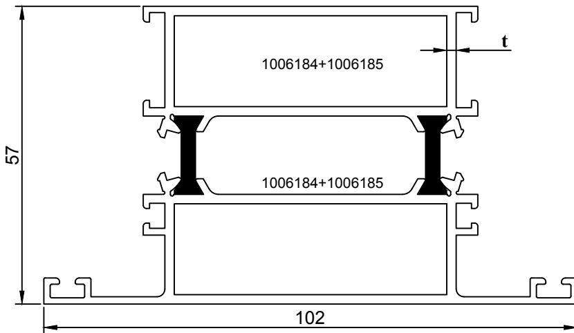
GENİŞ ORTA KAYIT PROFİLİ
