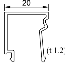
Profil No: 510676 Ağırlık : 0.216 Kg/m
