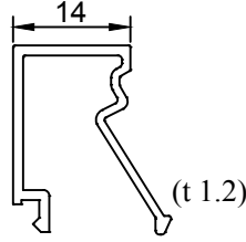
Profil No: 510692 Ağırlık : 0.197 Kg/m
