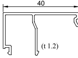
Profil No: 510685 Ağırlık : 0.300 Kg/m
