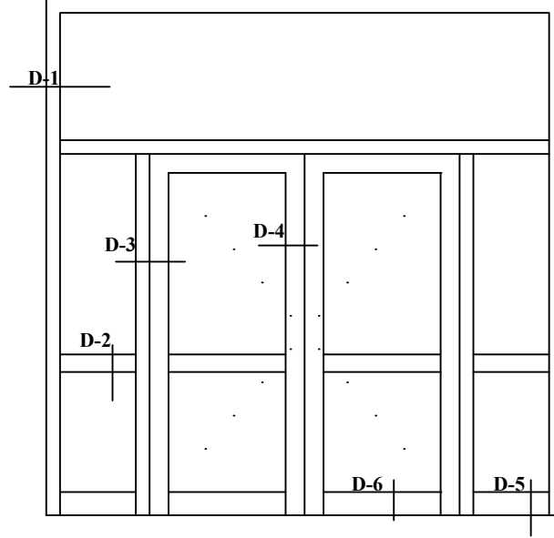
İÇE AÇILAN KAPILARDA ADAPTÖR UYGULAMASI
