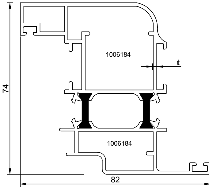
PVC AKSESURLARI UY.PROFİL
