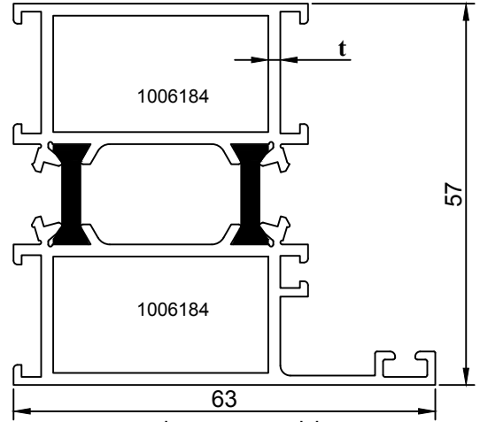
GENİŞ KASA PROFİLİ
