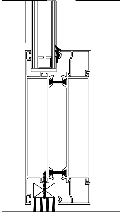
DETAY 6 KAPI ETEK DETAYI
