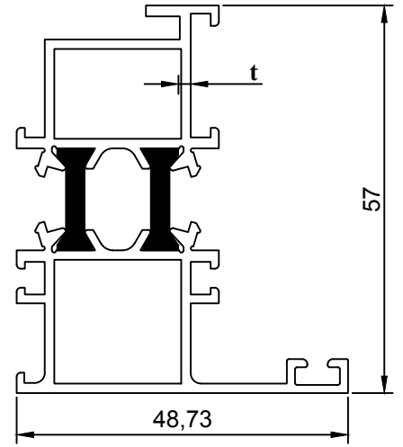
DIŞ KAPI ADAPTÖRÜ
