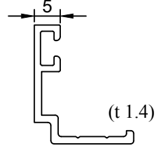
Profil No: 500691 Ağırlık : 0.186 Kg/m
