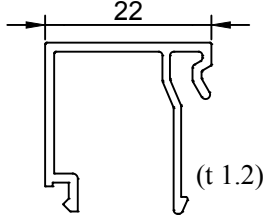
Profil No: 510629 Ağırlık : 0.240 Kg/m
