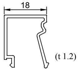
Profil No: 510674 Ağırlık : 0.211 Kg/m
