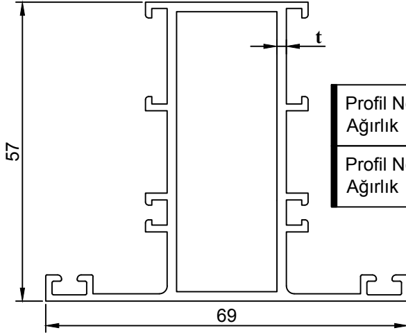
DAR ORTA KAYIT
