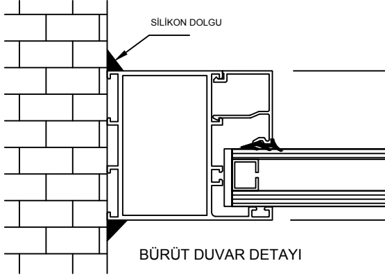
DETAY 1
