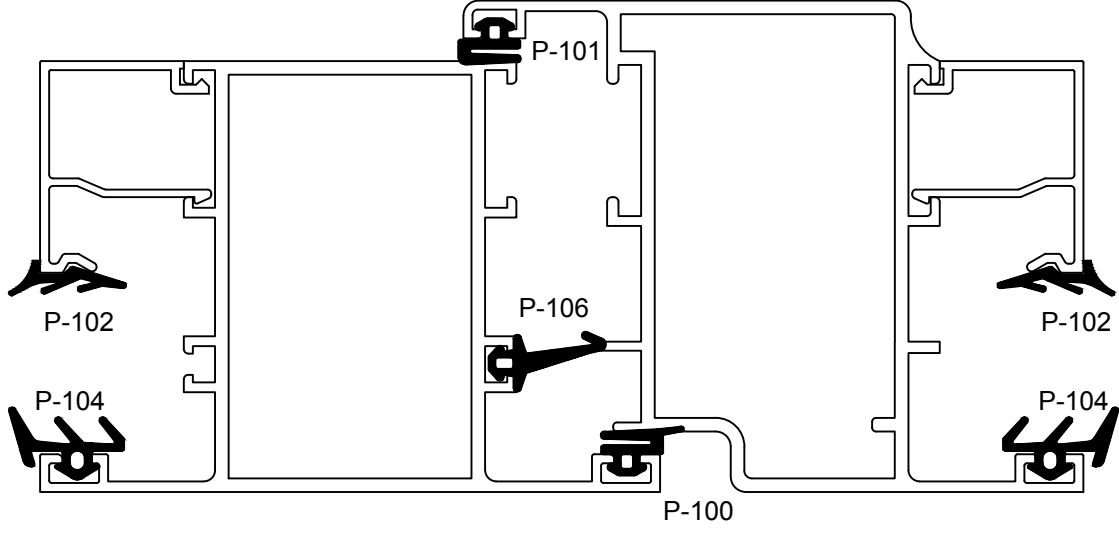
PENCERE FİTİL UYGULAMA DETAYI
