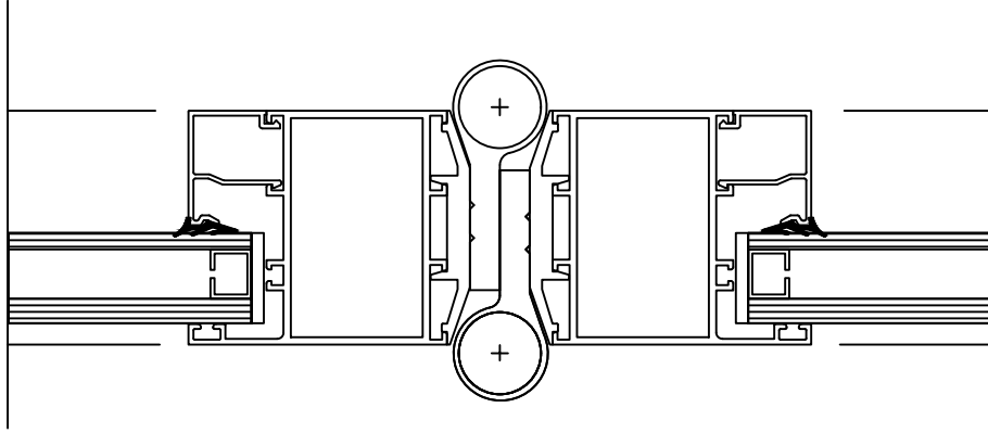
DETAY 20 ÇARPMA KAPI MENTEŞE DETAYI
