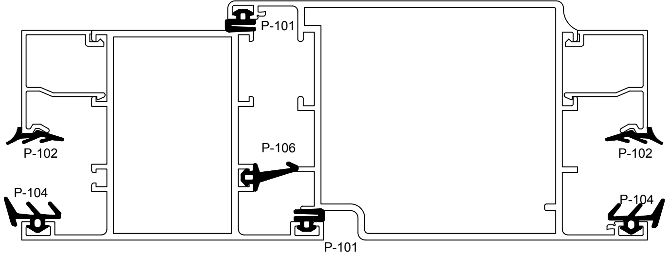
KAPI FİTİL UYGULAMA DETAYI
