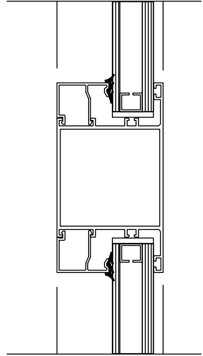
DETAY 2
