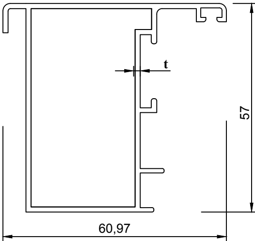
PİVOT ADAPTÖR PROFİLİ
