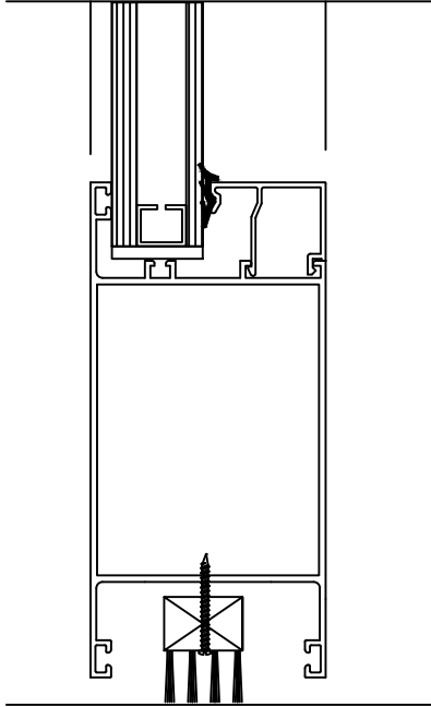
DETAY 22 KAPI ETEK DETAYI
