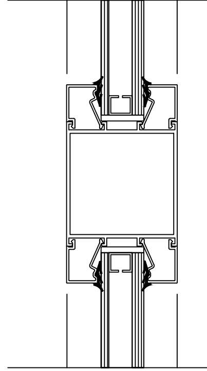
DETAY 15
