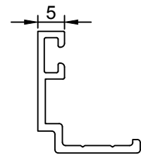
(t 1.4) 0.186 gr/m 500691
