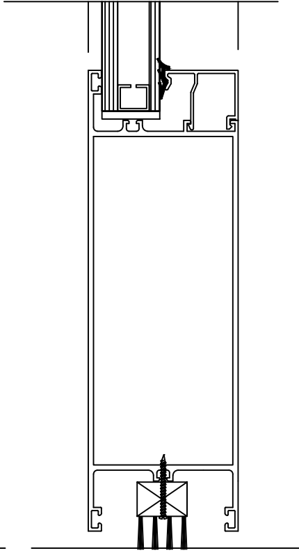
DETAY 6-A KAPI ETEK DETAYI
