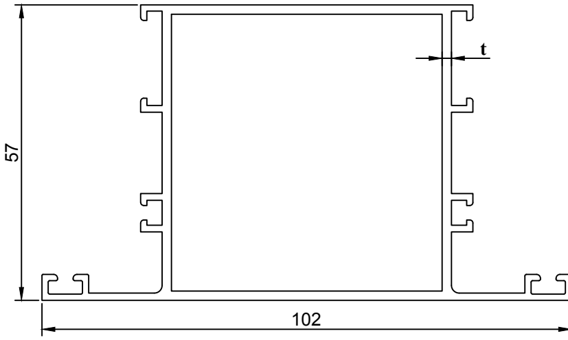
GENİŞ ORTA KAYIT
