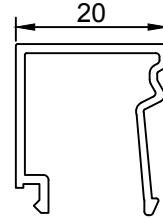
(t 1.2) 0.216 gr/m 510676
