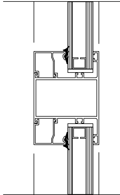
DETAY 11 ORTA KAYIT DETAYI
