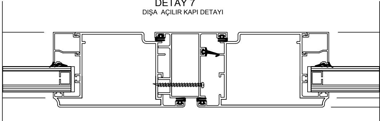
DETAY 8 DIŞA AÇILIR ÇİFT KAPI DETAYI
