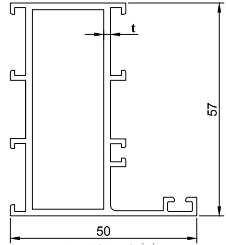
DAR KASA PROFİLİ
