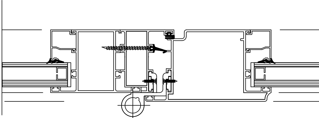
DETAY 7 DIŞA AÇILIR KAPI DETAYI
