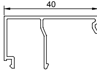
(t 1.2) 0.300 gr/m 500685
