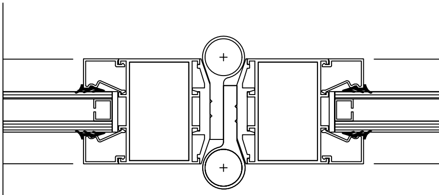
DETAY 16
