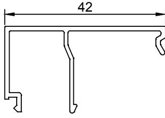
(t 1.2) 0.305 gr/m 510677
