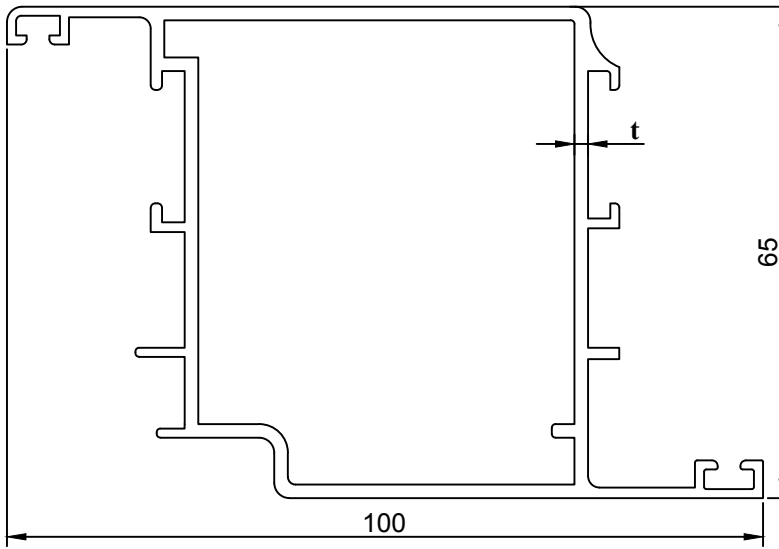
DAR İÇ KAPI PROFİLİ
