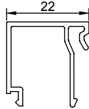
(t 1.2) 0.240 gr/m 510629
