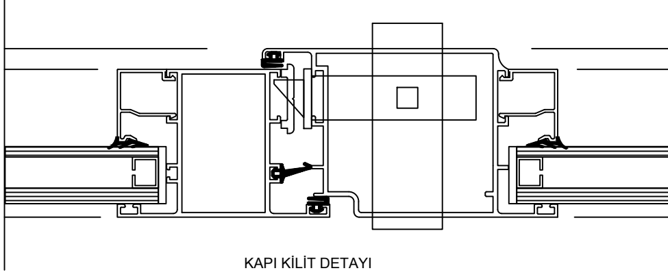
KAPI KİLİT DETAYI
