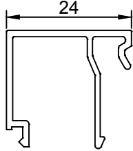
(t 1.2) 0.246 gr/m 510675
