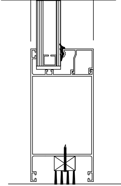
DETAY 6 KAPI ETEK DETAYI
