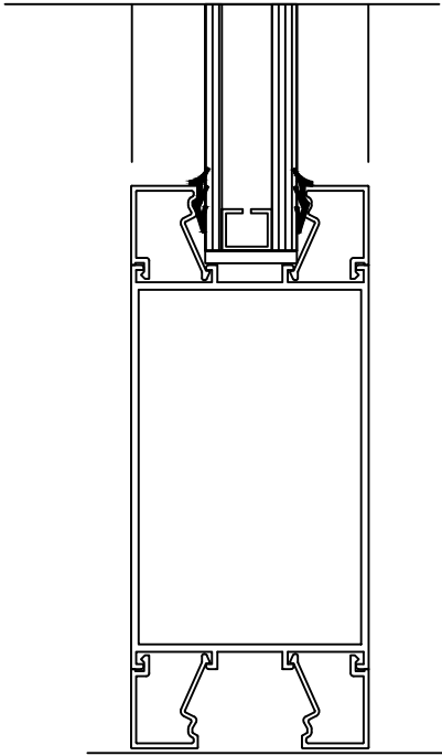
DETAY 18
