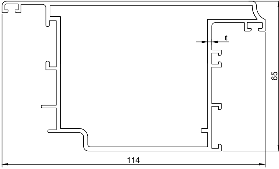
DIŞA AÇILIR KAPI PROFİLİ
