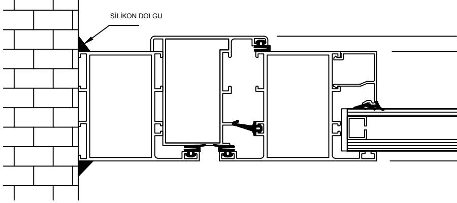
DETAY 12 PİVOT ADAPTÖR DETAYI
