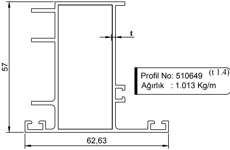
ÇİFT KAPI ADAPTÖRÜ
