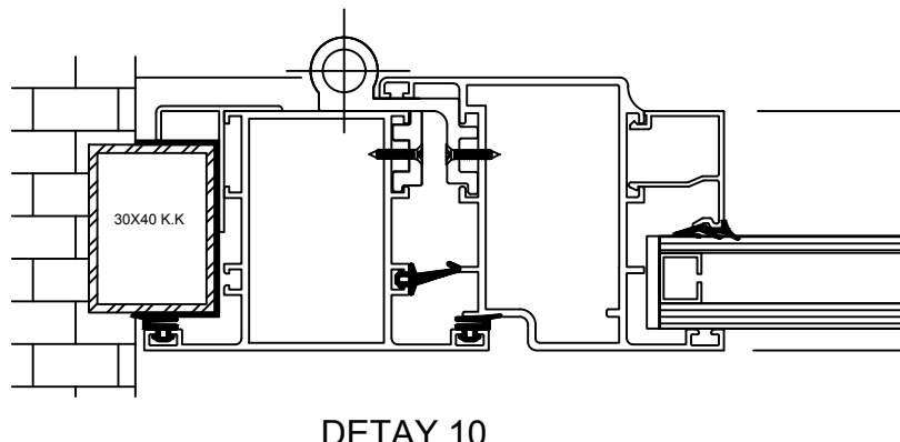
DETAY 10 PENCERE KANAT DETAYI
