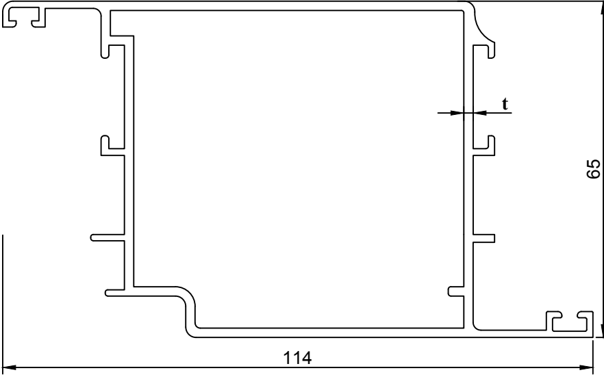
GENİŞ İÇ KAPI PROFİLİ
