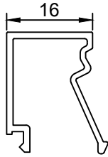
(t 1.2) 0.208 gr/m 500686
