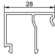
(t 1.2) 0.262 gr/m 500651
