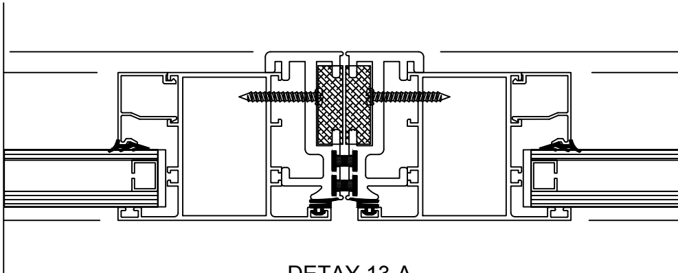
DETAY 13-A PİVOT MENTEŞE DETAYI
