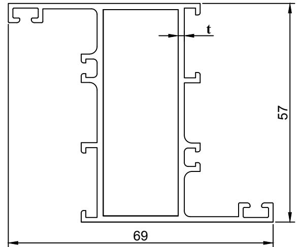
Z KASA PROFİLİ
