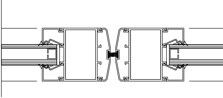
DETAY 17
