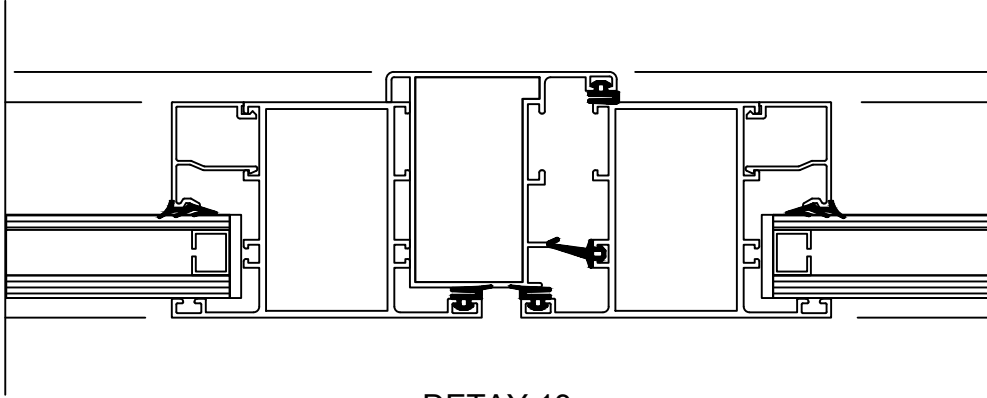
DETAY 13 PİVOT ADAPTÖR DETAYI
