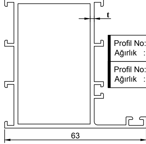
KASA PROFİLİ
