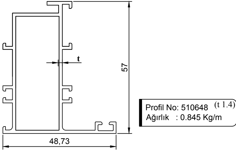
DIŞ KAPI ADAPTÖRÜ
