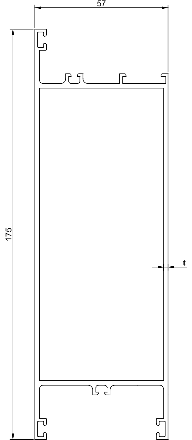
175 LİK ETEK
