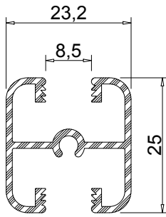
Profil No: 550630 Ağırlık: 0,370 Kg/m
