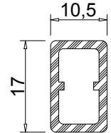
Profil No: 1006124 Ağırlık: 0,220 Kg/m
