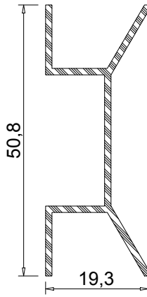
Profil No: 430690 Ağırlık: 0,327 Kg/m
