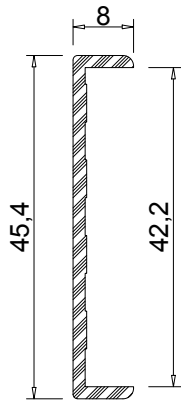
Profil No: 560632 Ağırlık: 0,270 Kg/m
