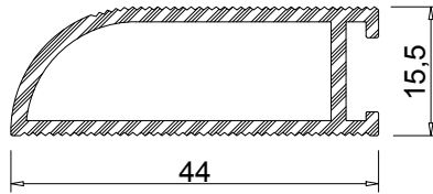
Profil No: 1006190 Ağırlık: 0,510 Kg/m
