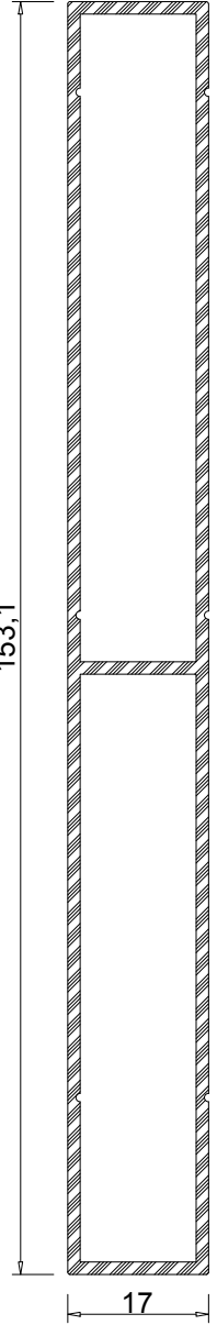
Profil No: 490630 Ağırlık: 1,410 Kg/m
