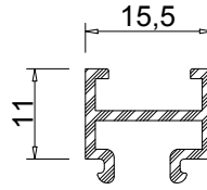
Profil No: 1406597 Ağırlık: 0,175 Kg/m
