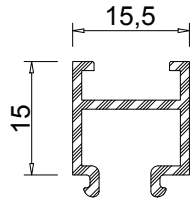
Profil No: 1006298 Ağırlık: 0,200 Kg/m
