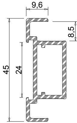
Profil No: 1006217 Ağırlık: 0,500 Kg/m
