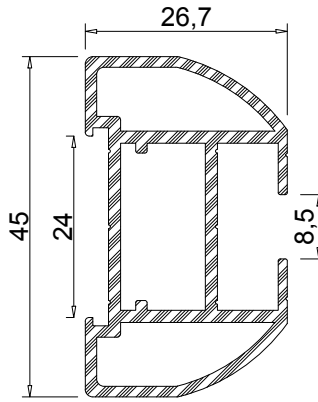
Profil No: 1006228 Ağırlık: 0,800 Kg/m
