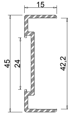
Profil No: 1506549 Ağırlık: 0,330 Kg/m
