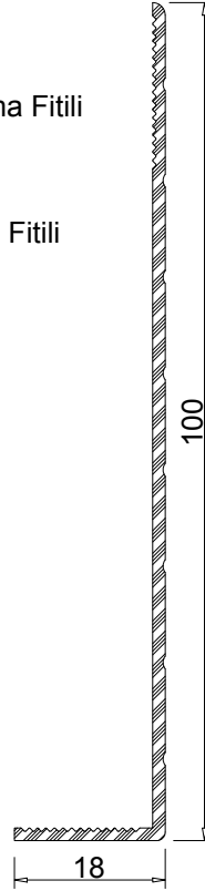
Profil No: 1006129 Ağırlık: 0,500 Kg/m
