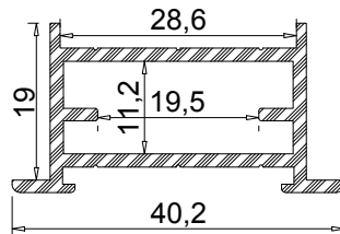
Profil No : 640640 Ağırlık : 0,485 Kg/m
