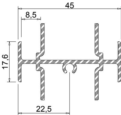
Profil No: 1006227 Ağırlık: 0,625 Kg/m
