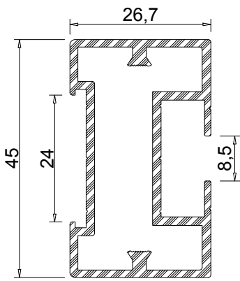
Profil No: 1406577 Ağırlık: 0,800 Kg/m
