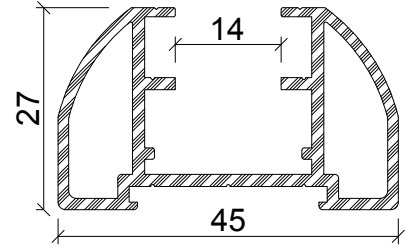
Profil No : 1506518 Ağırlık : 0,690 Kg/m
