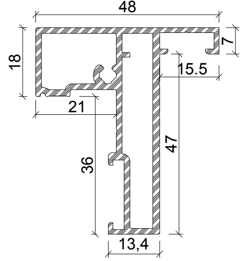
Profil No : 750678 Ağırlık : 0,944 Kg/m
