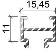
Profil No: 1406597 Ağırlık: 0,175 Kg/m
