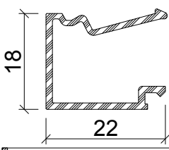
Profil No : 510674 Ağırlık : 0,211 Kg/m
