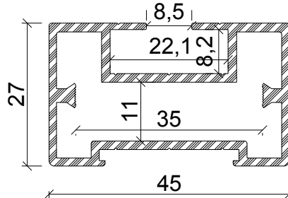
Profil No : 1406577 Ağırlık : 0,800 Kg/m
