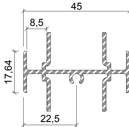
Profil No : 1006227 Ağırlık : 0,625 Kg/m
