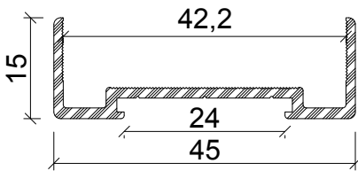
Profil No : 1506549 Ağırlık : 0,330 Kg/m
