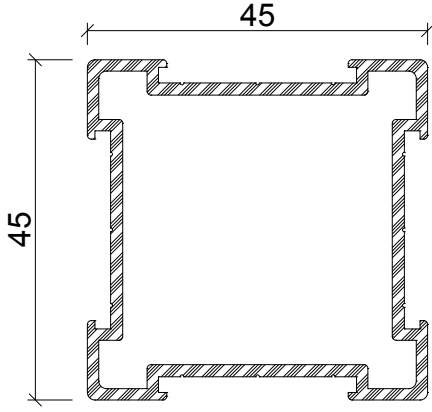
Profil No: 1006226 Ağırlık: 0,853 Kg/m
