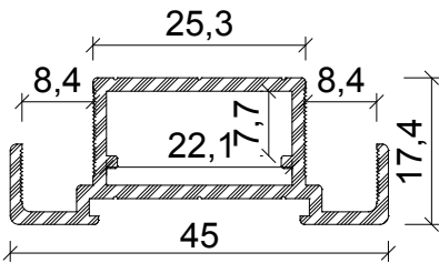
Profil No : 1006217 Ağırlık : 0,500 Kg/m
