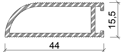
Profil No : 1006190 Ağırlık : 0,510 Kg/m
