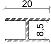
Profil No: 580688 Ağırlık: 0,145 Kg/m
