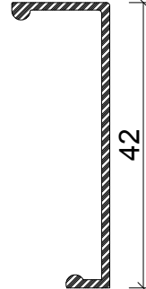
Profil No : 770690 Ağırlık : 0,205 Kg/m
