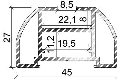
Profil No : 1006228 Ağırlık : 0,800 Kg/m
