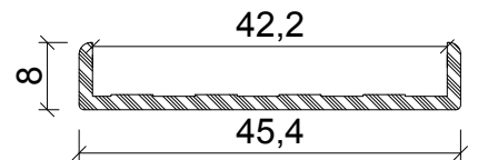
Profil No : 560632 Ağırlık : 0,270 Kg/m
