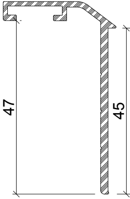
Profil No : 440682 Ağırlık : 0,415 Kg/m
