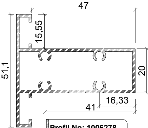
Profil No : 1006278 Ağırlık : 0,810 Kg/m
