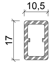
Profil No: 1006124 Ağırlık : 0,220 Kg/m
