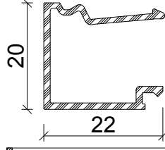
Profil No : 510676 Ağırlık : 0,216 Kg/m
