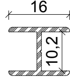
Profil No: 570626 Ağırlık: 0,135 Kg/m
