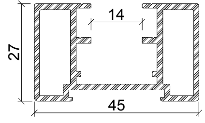
Profil No : 1506519 Ağırlık : 0,745 Kg/m
