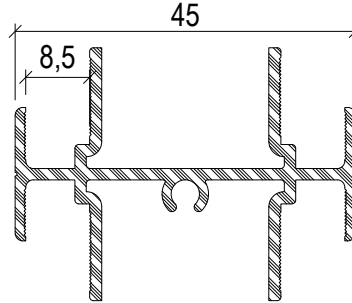
Profil No : 1006227 Ağırlık : 0,620 Kg/m
