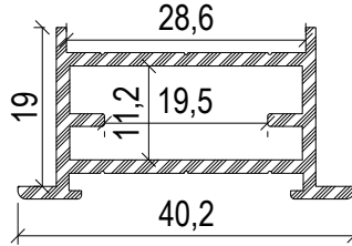
Profil No : 640640 Ağırlık : 0,490 Kg/m
