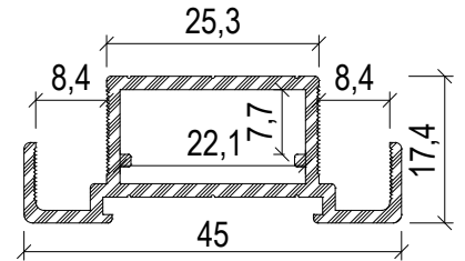
Profil No : 1006217 Ağırlık : 0,500 Kg/m
