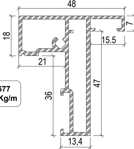
Profil No : 750678 Ağırlık : 0,945 Kg/m
