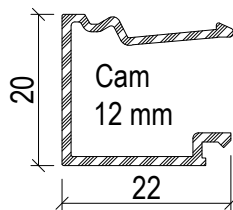
Profil No : 510676 Ağırlık : 0,220 Kg/m
