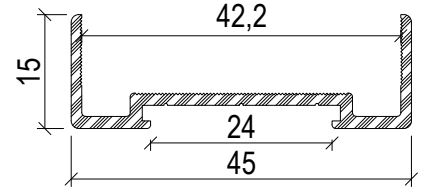
Profil No : 1506549 Ağırlık : 0,330 Kg/m
