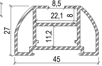
Profil No : 1006228 Ağırlık : 0,800 Kg/m
