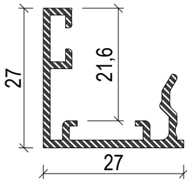
Profil No : 750676 Ağırlık : 0,330 Kg/m
