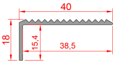
Profil No : 180677 Ağırlık : 0,260 Kg/m
