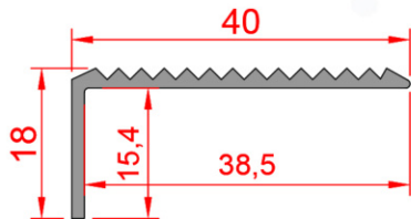
Profil No : 180677 Ağırlık : 0,260 Kg/m
