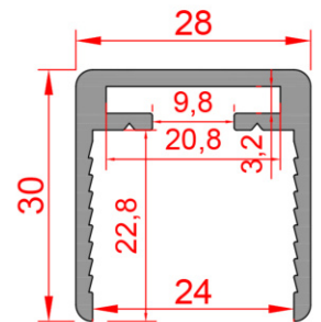
Profil No : 760690 Ağırlık : 0,530 Kg/m
