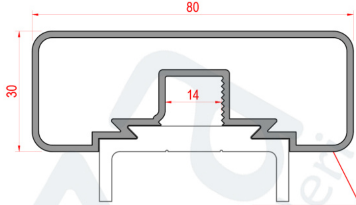
Profil No : 640646 Ağırlık : 1,095 Kg/m
