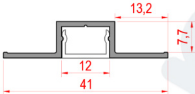
Profil No : 1006220 Ağırlık : 0,195 Kg/m
