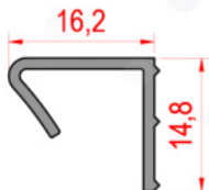
Profil No : 1006481 Ağırlık : 0,130 Kg/m
