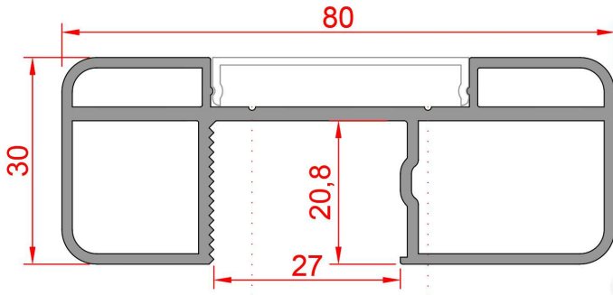
Profil No : 1006400 Ağırlık : 1,210 Kg/m
