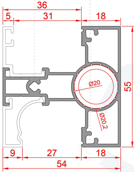
Profil No : 1006401 Ağırlık : 1,050 Kg/m
