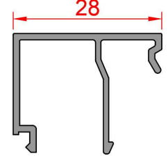
Profil No : 500651 Ağırlık : 0,260 Kg/m
