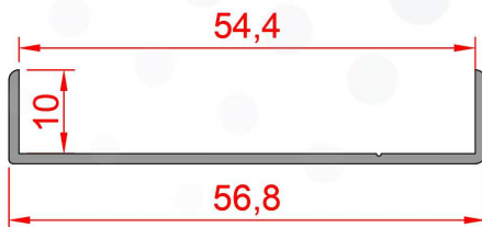
Profil No : 1006402 Ağırlık : 0,250 Kg/m
