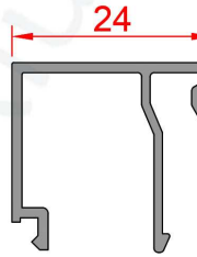
Profil No : 510675 Ağırlık : 0,250 Kg/m
