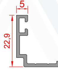
Profil No : 500691 Ağırlık : 0,190 Kg/m
