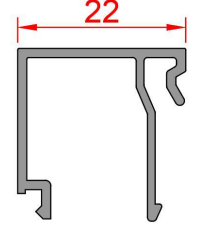
Profil No : 510629 Ağırlık : 0,240 Kg/m
