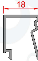
Profil No : 510674 Ağırlık : 0,220 Kg/m
