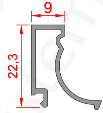
Profil No : 1006115 Ağırlık : 0,200 Kg/m
