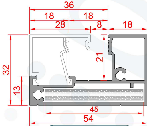
Profil No : 370690 Ağırlık : 0,770 Kg/m
