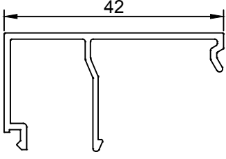
Profil No: 510677 (t 1.2) Ağırlık : 0.305 Kg/m
