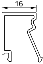
Profil No: 510686 (t 1.2) Ağırlık : 0.208 Kg/m
