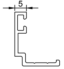
Profil No: 500691 (t 1.4) Ağırlık : 0.186 Kg/m
