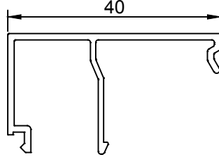
Profil No: 510685 (t 1.2) Ağırlık : 0.300 Kg/m
