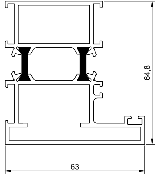
Profil No: 1006135 (t 1.8) Ağırlık : 1.916 Kg/m
