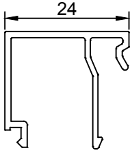
Profil No: 510675 (t 1.2) Ağırlık : 0.246 Kg/m
