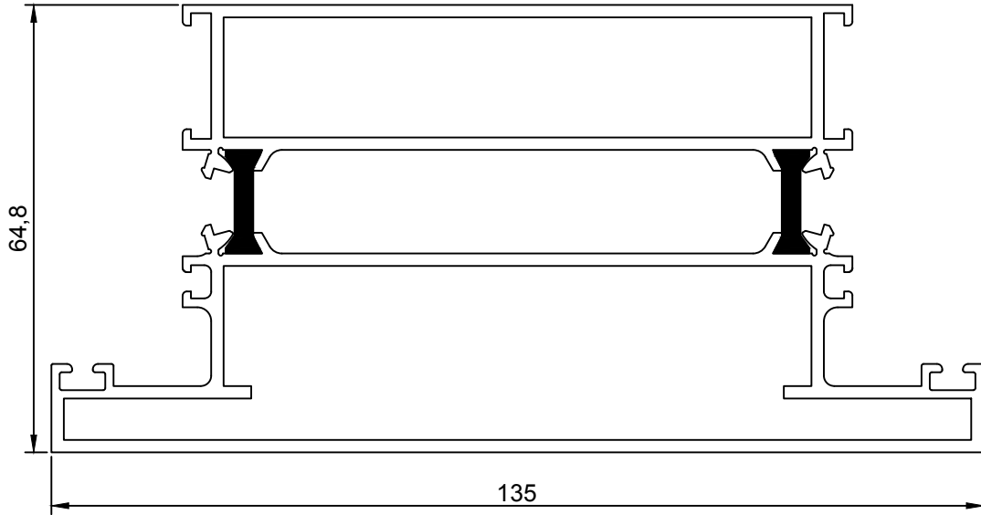
Profil No: 1006156 (t 1.8) Ağırlık : 3.094 Kg/m
