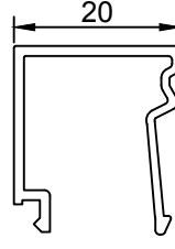
Profil No: 510676 (t 1.2) Ağırlık : 0.216 Kg/m
