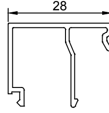
Profil No: 500651 (t 1.2) Ağırlık : 0.262 Kg/m
