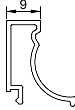
Profil No: 1006155 (t 1.2) Ağırlık : 0.197 Kg/m
