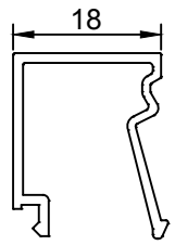
Profil No: 510674 (t 1.2) Ağırlık : 0.211 Kg/m
