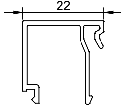
Profil No: 510629 (t 1.2) Ağırlık : 0.240 Kg/m
