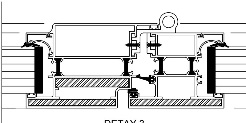
DETAY 3 İÇ KAPI DETAYI
