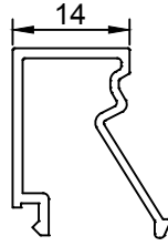
Profil No: 510692 (t 1.2) Ağırlık : 0.197 Kg/m
