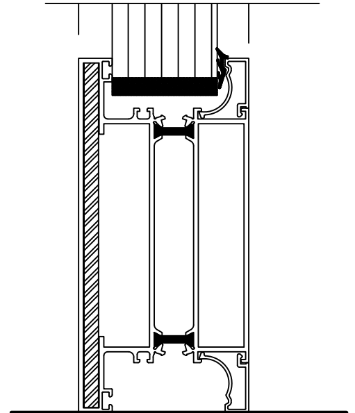
DETAY 4 ETEK DETAYI
