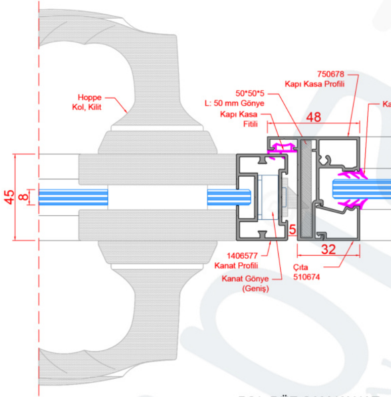
D21_DÜZ CAM KANAT + KAPI KASA SABİT CAM DETAYI
