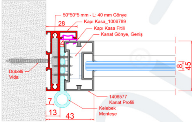
D28_DAR KAPI KASA, DÜZ CAM KANAT DETAYI 2
