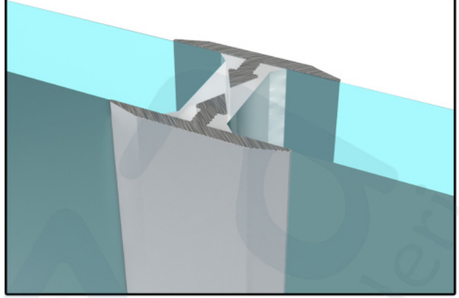
D65_15 MM T PROFİLİ İLE 10 MM CAM CAMA BİRLEŞİM DETAYI
