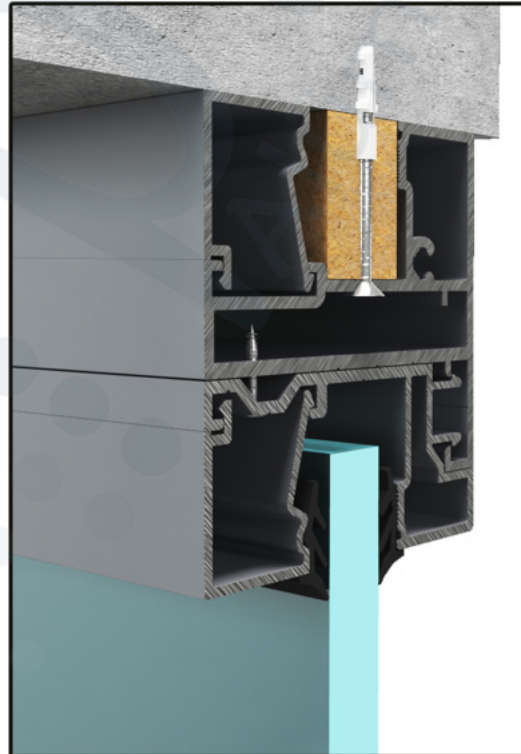
D42_KANAT ÜSTÜ - SABİT CAM DETAYI 3 - DİKEY KESİT
