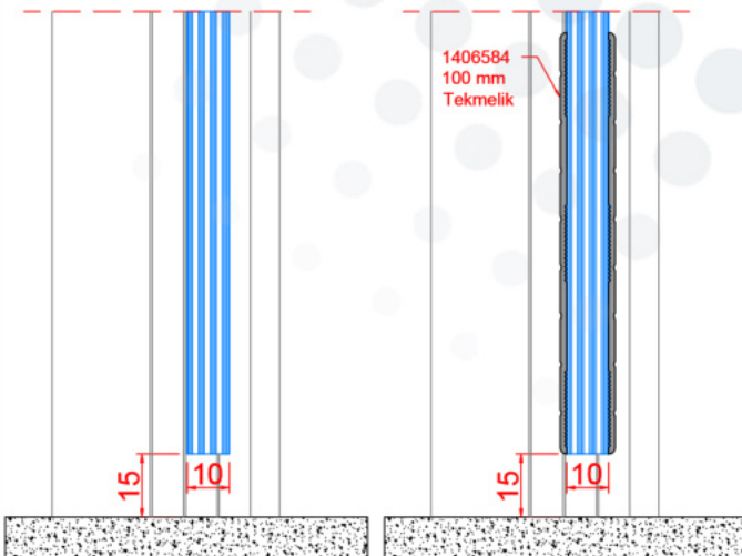
D12_10 MM CAM KANAT ALT DETAYLARI
