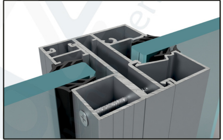
D36_KANAT ÜSTÜ - SABİT CAM DETAYI 1 - YATAY KESİT
