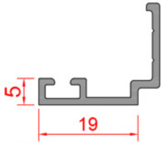
Profil No: 500691 Ağırlık: 0,190 Kg/m
