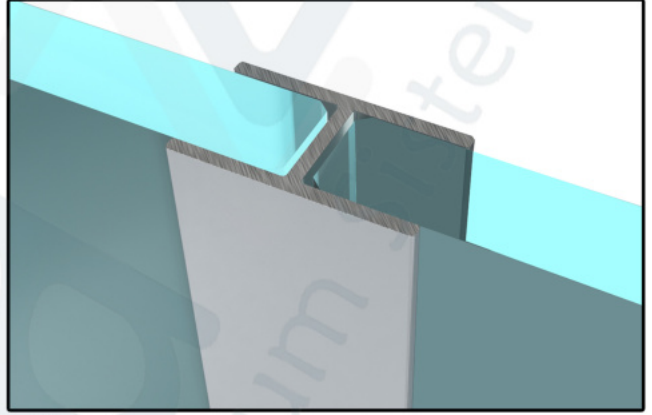
D70_8 MM CAM, H PROFİLİ İLE CAM CAMA BİRLEŞİM DETAYI
