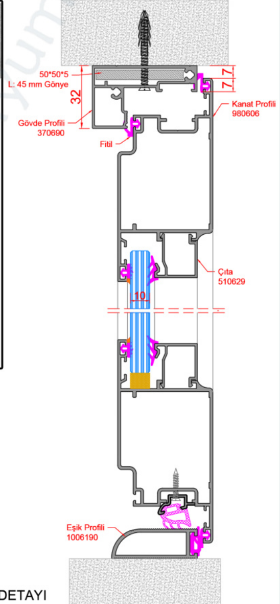
D45_ORTA KAYIT PROFİLİNE + AÇILIR SİSTEM KANAT DETAYI
