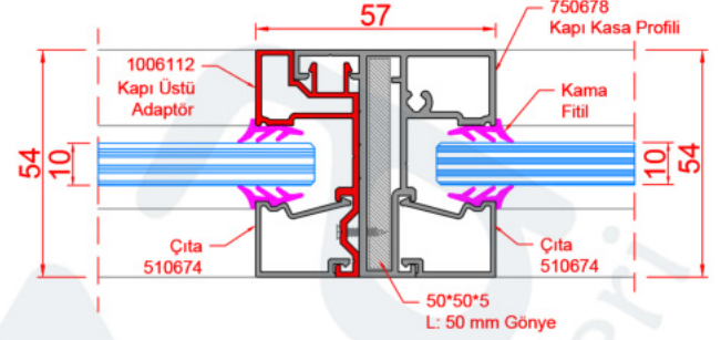
D41_KAPI KASA PROFİLİ + KANAT ÜSTÜ SABİT CAM ADAPTÖR PROFİLİ DETAYI
