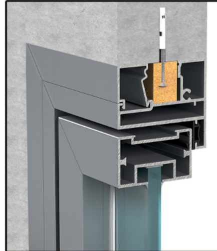
D22_TAVAN KAPI KASA + DÜZ CAM KANAT DETAYI
