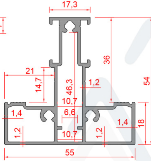
Profil No : 370691 Ağırlık : 1,030 Kg/m
