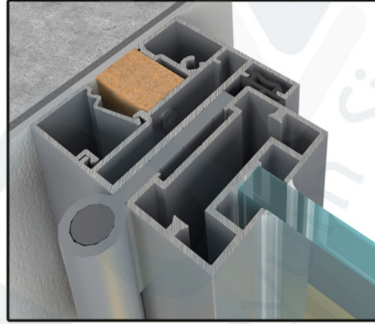
D18_KAPI KASA + DÜZ CAM KANAT DETAYI
