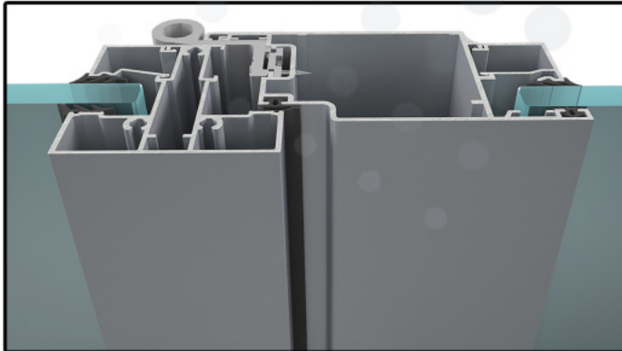
D44_SABİT CAMLI ORTA KAYIT PROFİLİNE + AÇILIR SİSTEM KANAT DETAYI
