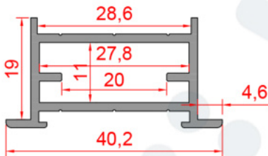
Profil No : 640640 Ağırlık : 0,490 Kg/m
