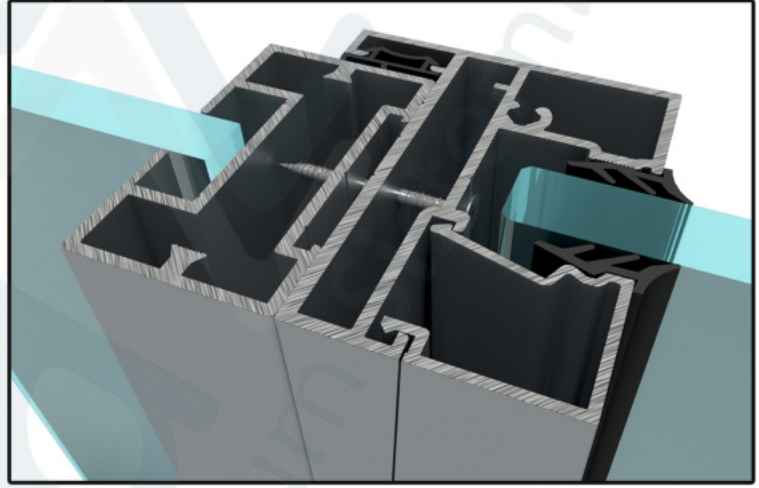
D38_KANAT ÜSTÜ - SABİT CAM DETAYI 2 - YATAY KESİT
