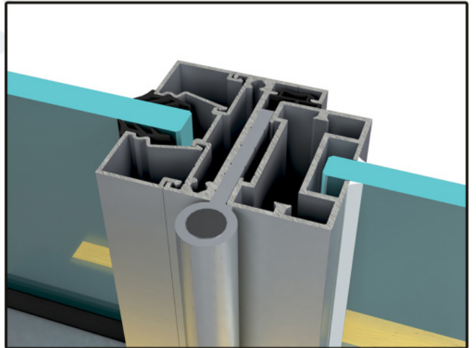
D29_SABİT CAMLI, DAR KAPI KASA + DÜZ CAM KANAT DETAYI
