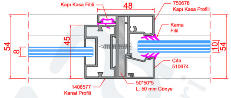
D38_KANAT ÜSTÜ - SABİT CAM DETAYI 2 - YATAY KESİT
