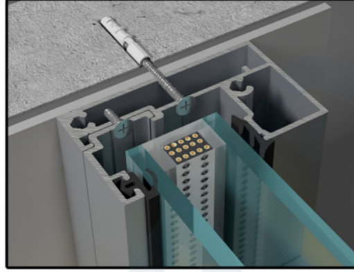
D17_KASA PROFİLİNE - 4+16+4 ISICAM DETAYI
