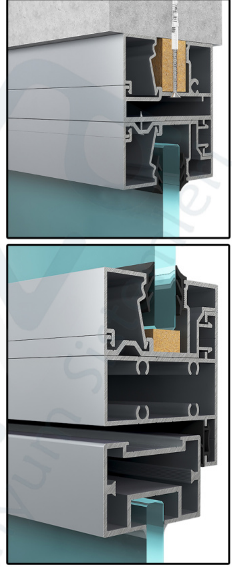
D43_KANAT ÜSTÜ, T PROFİLİ VE ADAPTÖRLÜ - SABİT CAM DETAYI - DİKEY KESİT
