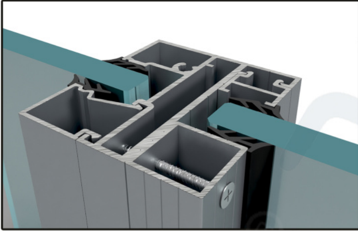
D36_KANAT ÜSTÜ - SABİT CAM DETAYI 1 - YATAY KESİT
