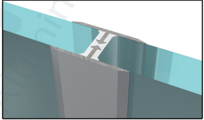
D67_25 MM T PROFİLİ İLE 12 MM CAM CAMA BİRLEŞİM DETAYI
