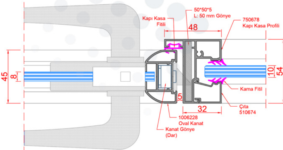
D50_OVAL CAM KANAT + SABİT CAMLI KAPI KASA DETAYI
