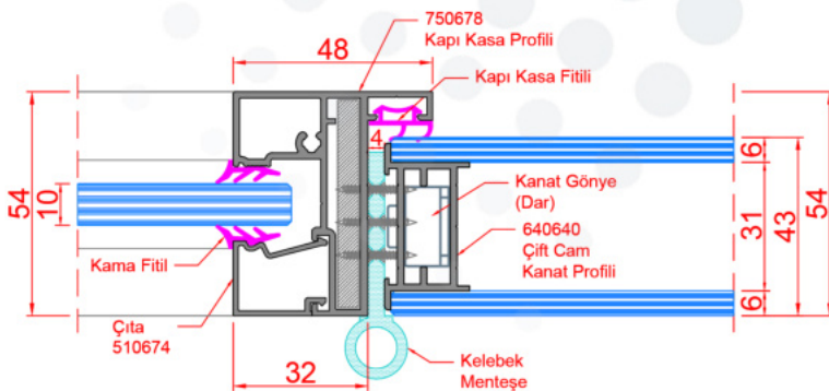
D57_SABİT CAMLI KAPI KASA + ÇİFT YÜZ CAM KANAT DETAYI
