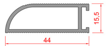
Profil No : 1006190 Ağırlık : 0,510 Kg/m
