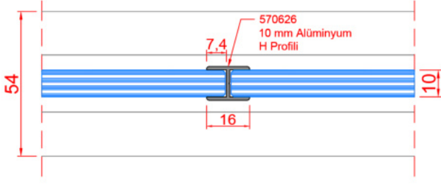
D69_10 MM CAM, H PROFİLİ İLE CAM CAMA BİRLEŞİM DETAYI
