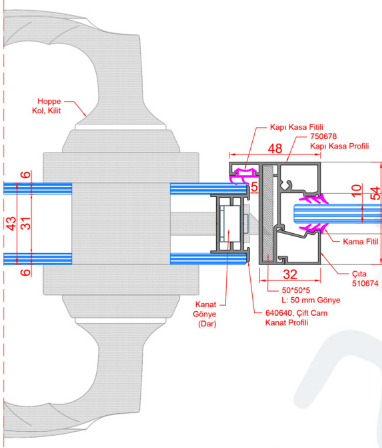
D58_ÇİFT YÜZ CAM KANAT + SABİT CAMLI KAPI KASA DETAYI
