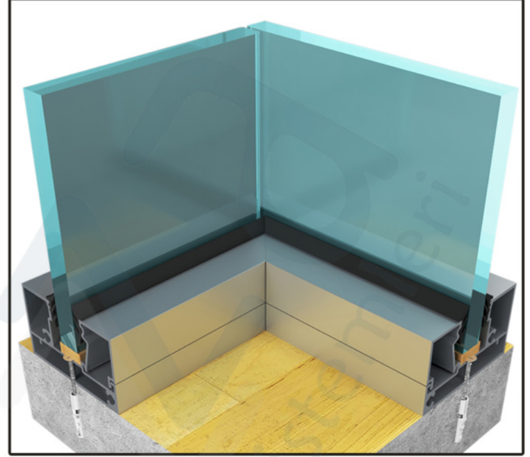
D13_10 MM CAM CAMA - 90° KÖŞE BİRLEŞİM DETAYI
