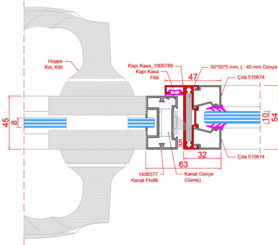
D31_DÜZ CAM KANAT + KAPI KASA YENİ, SABİT CAM DETAYI
