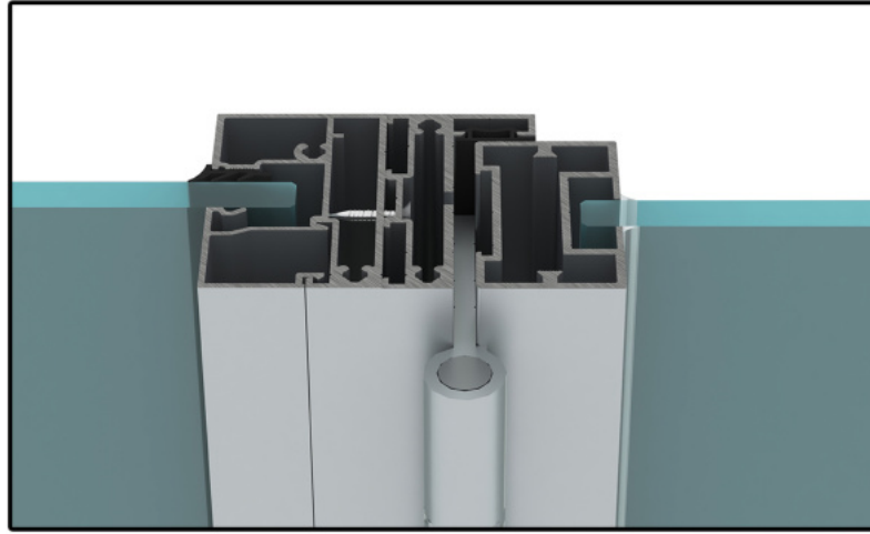
D30_GÖVDE PROFİLİ VE KAPI KASA PROFİLİ DETAYI
