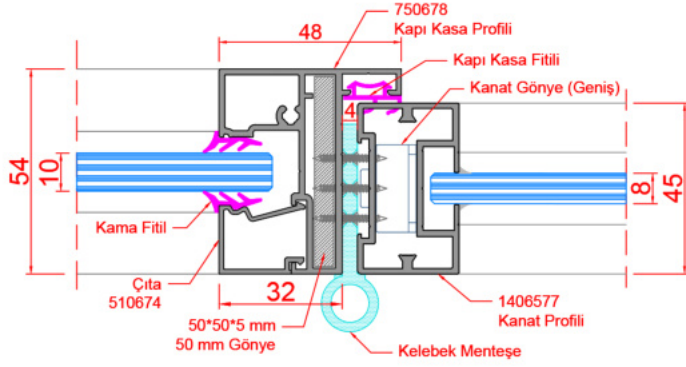
D20_SABİT CAMLI KAPI KASA + DÜZ CAM KANAT DETAYI
