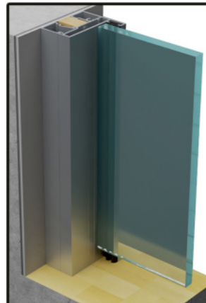
D12_10 MM CAM KANAT ALT DETAYLARI
