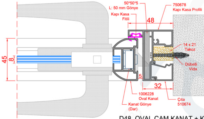
D48_OVAL CAM KANAT + KAPI KASA DETAYI
