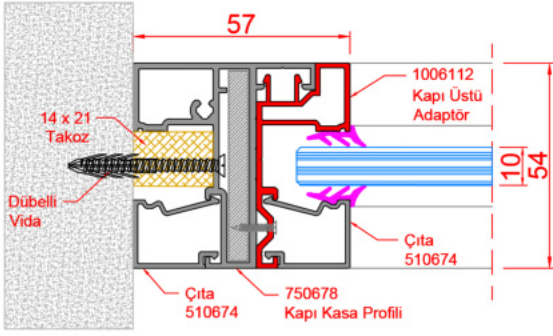
D40_DUVARA KAPI KASA PROFİLİ + KANAT ÜSTÜ SABİT CAM, ADAPTÖR PROFİL DETAYI
