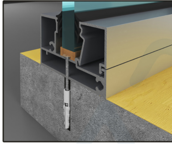
D1_ZEMİN DETAYI 1
