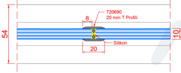
D66_20 MM T PROFİLİ İLE 10 MM CAM CAMA BİRLEŞİM DETAYI
