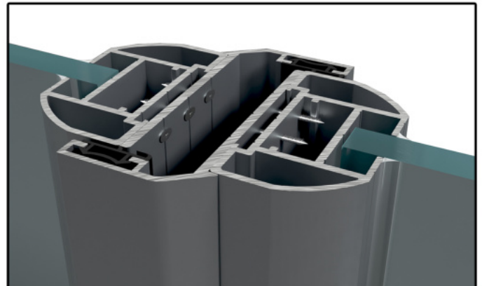
D54_OVAL CAM KANAT, ÇİFT KANAT DETAYI
