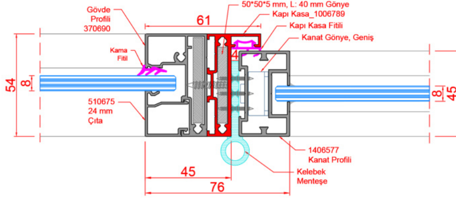
D30_GÖVDE PROFİLİ VE KAPI KASA PROFİLİ DETAYI
