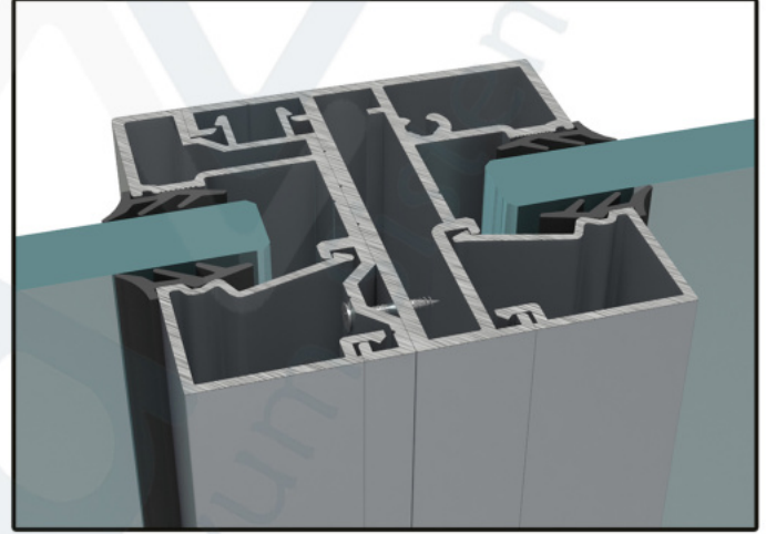
D41_KAPI KASA PROFİLİ + KANAT ÜSTÜ SABİT CAM ADAPTÖR PROFİLİ DETAYI
