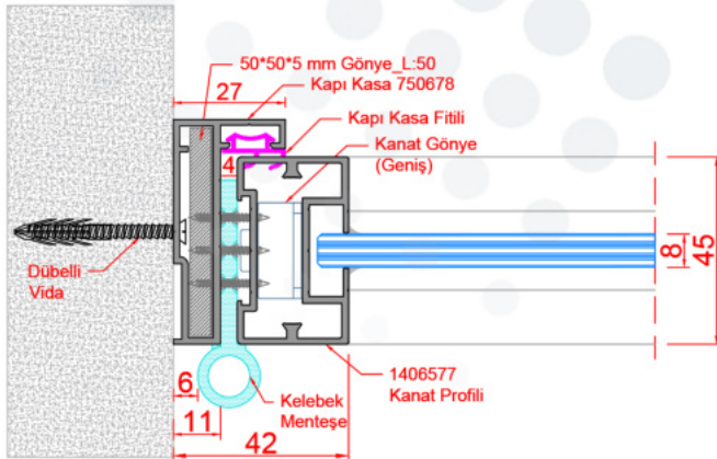
D26_DAR KAPI KASA, DÜZ CAM KANAT DETAYI 1
