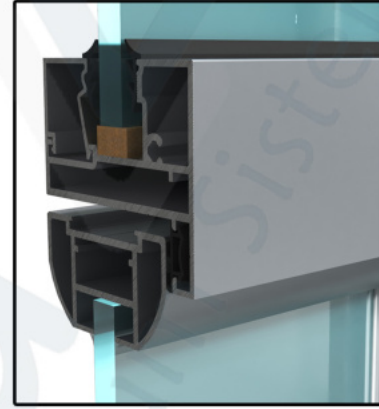
D52_OVAL CAM KANAT ÜSTÜ + KAPI KASA DETAYI
