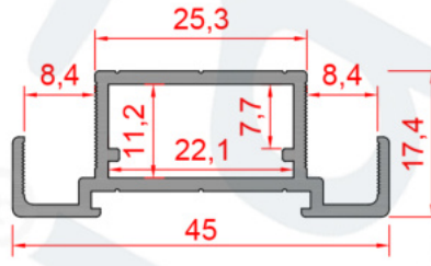
Profil No : 1006217 Ağırlık : 0,500 Kg/m
