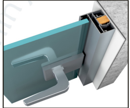
D6_DUVAR - 10 MM CAM KAPI KANAT + PIAZZA MENTEŞE DETAYI
