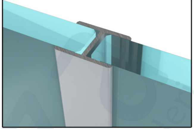
D69_10 MM CAM, H PROFİLİ İLE CAM CAMA BİRLEŞİM DETAYI
