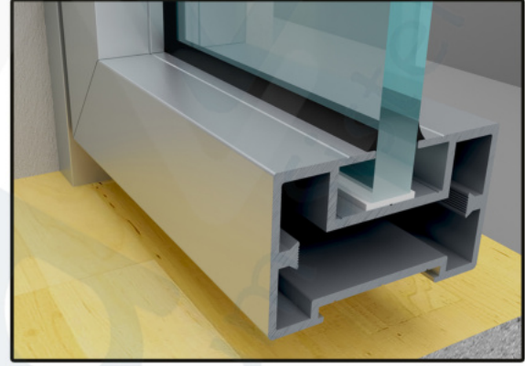
D24_DÜZ CAM KANAT ZEMİN DETAYI
