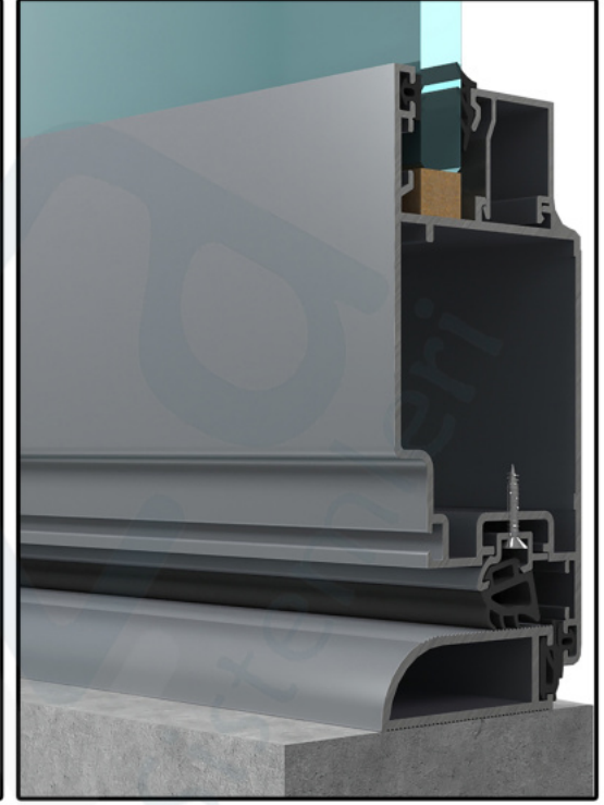
D45_ORTA KAYIT PROFİLİNE + AÇILIR SİSTEM KANAT DETAYI
