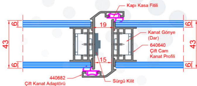
D62_ÇİFT YÜZ CAM KANAT, ÇİFT KANAT DETAYI
