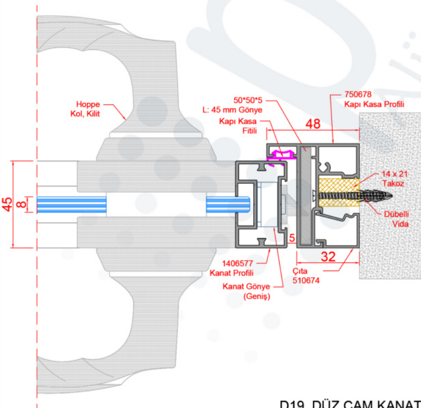
D19_DÜZ CAM KANAT + KAPI KASA DETAYI
