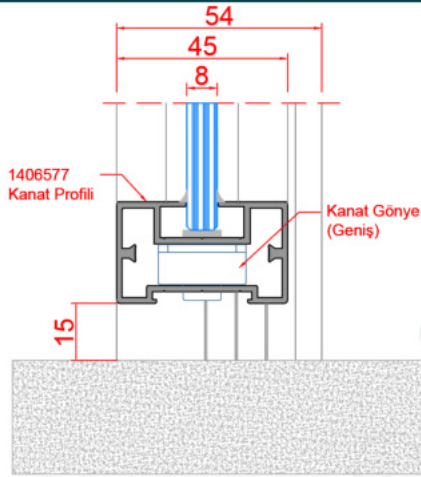
D24_DÜZ CAM KANAT ZEMİN DETAYI
