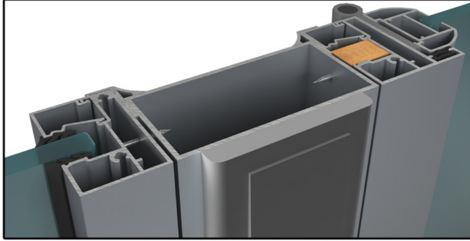
D15_TEKNİK PANEL DETAYI - 45*90 KUTU PROFİLİ
