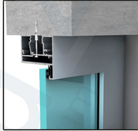
D10_TAVAN + 10 MM CAM KANAT DETAYI
