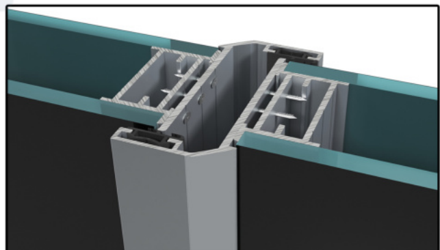
D62_ÇİFT YÜZ CAM KANAT, ÇİFT KANAT DETAYI
