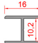
Profil No: 570626 Ağırlık: 0,140 Kg/m
