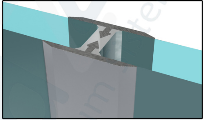
D66_20 MM T PROFİLİ İLE 10 MM CAM CAMA BİRLEŞİM DETAYI
