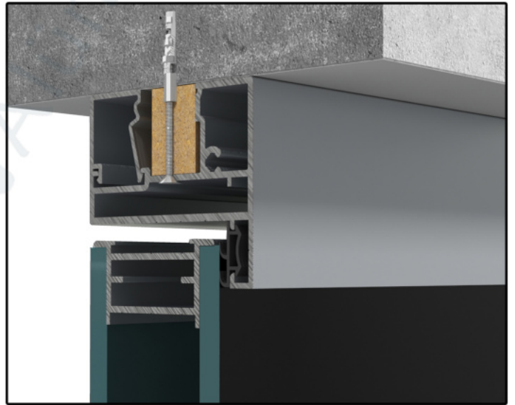
D59_TAVAN KAPI KASA + ÇİFT YÜZ CAM KANAT DETAYI
