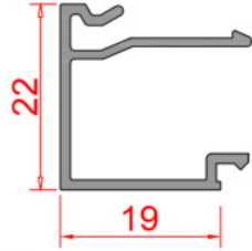
Profil No : 510629 Ağırlık : 0,240 Kg/m
