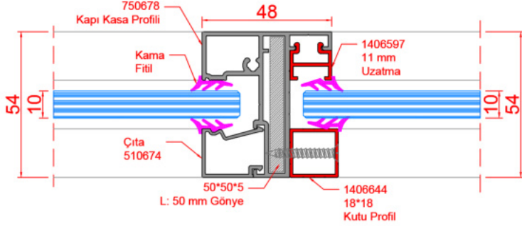
D36_KANAT ÜSTÜ - SABİT CAM DETAYI 1 - YATAY KESİT
