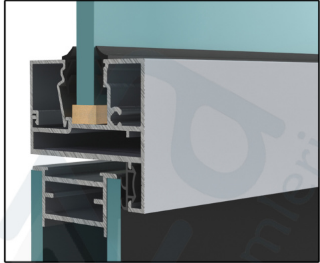
D60_ÇİFT YÜZ CAM KANAT ÜSTÜ + KAPI KASA DETAYI
