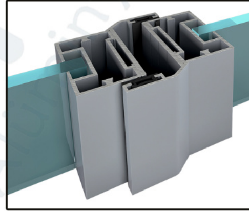
D25_DÜZ CAM KANAT, ÇİFT KANAT DETAYI
