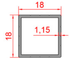
Profil No : 1406644 Ağırlık : 0,210 Kg/m
