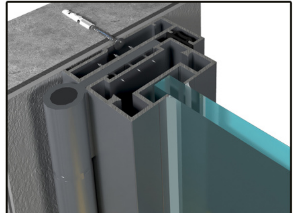
D26_DAR KAPI KASA, DÜZ CAM KANAT DETAYI 1
