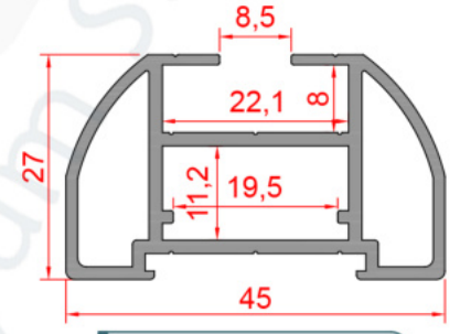
Profil No : 1006228 Ağırlık : 0,800 Kg/m
