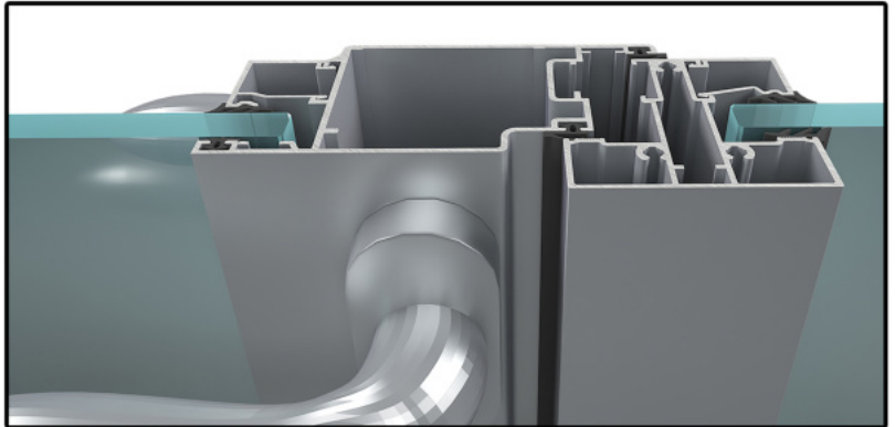
D44_SABİT CAMLI ORTA KAYIT PROFİLİNE + AÇILIR SİSTEM KANAT DETAYI
