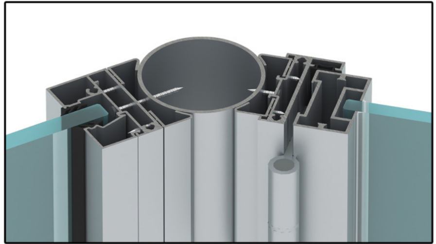
D32_Ø60 BORU PROFİLİ, AÇILI DÖNÜŞ SABİT CAM VE KANAT DETAYI 1
