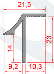
Profil No : 1006198 Ağırlık : 0,200 Kg/m
