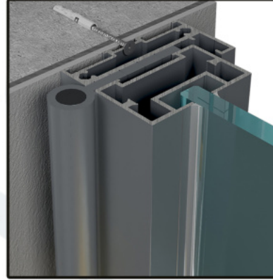
D28_DAR KAPI KASA, DÜZ CAM KANAT DETAYI 2
