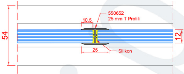
D67_25 MM T PROFİLİ İLE 12 MM CAM CAMA BİRLEŞİM DETAYI
