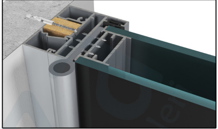
D55_KAPI KASA + ÇİFT YÜZ CAM KANAT DETAYI
