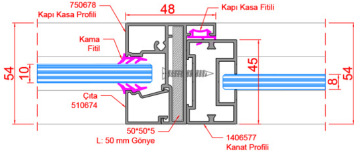
D38_KANAT ÜSTÜ - SABİT CAM DETAYI 2 - YATAY KESİT
