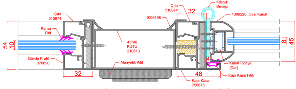
D15_TEKNİK PANEL DETAYI - 45*90 KUTU PROFİLİ
