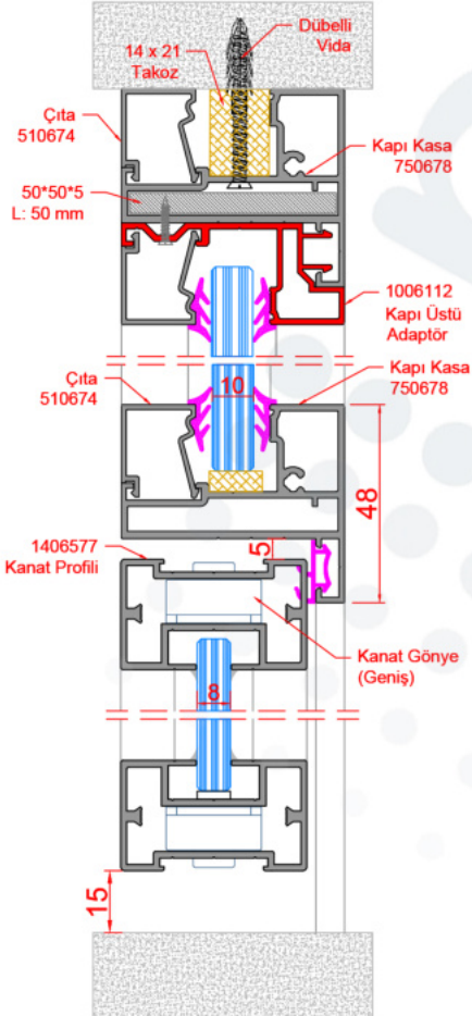
D42_KANAT ÜSTÜ - SABİT CAM DETAYI 3 - DİKEY KESİT
