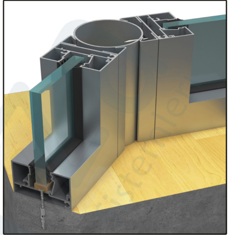
D34 _Ø60 BORU PROFİLİLE, AÇILI DÖNÜŞ DETAYI 1
