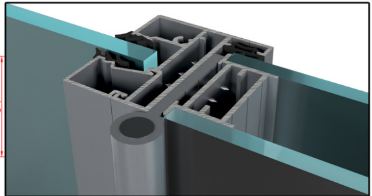
D57_SABİT CAMLI KAPI KASA + ÇİFT YÜZ CAM KANAT DETAYI
