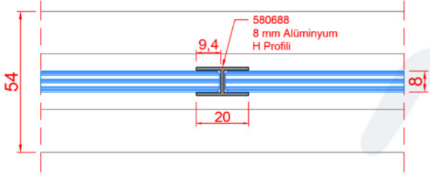
D70_8 MM CAM, H PROFİLİ İLE CAM CAMA BİRLEŞİM DETAYI
