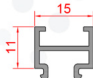
Profil No: 1406597 Ağırlık: 0,180 Kg/m
