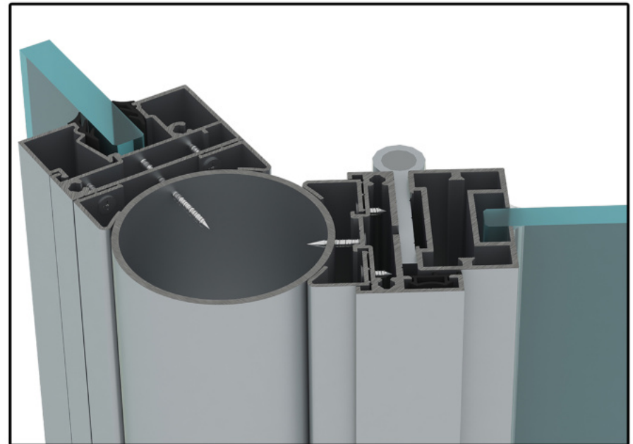
D33_Ø60 BORU PROFİLİ, AÇILI DÖNÜŞ SABİT CAM VE KANAT DETAYI 2
