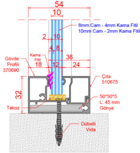
D27_ZEMİN DETAYI 2
