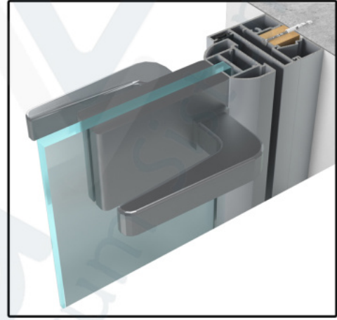
D48_OVAL CAM KANAT + KAPI KASA DETAYI
