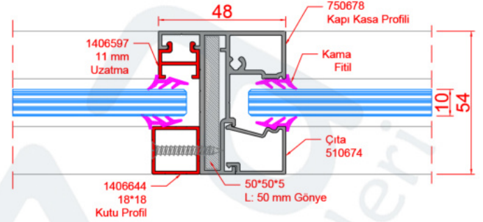
D36_KANAT ÜSTÜ - SABİT CAM DETAYI 1 - YATAY KESİT
