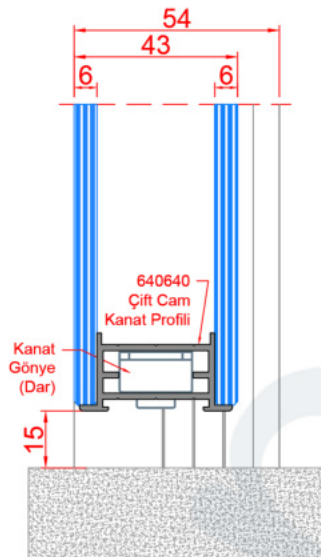
D61_ÇİFT YÜZ CAM KANAT ZEMİN DETAYI
