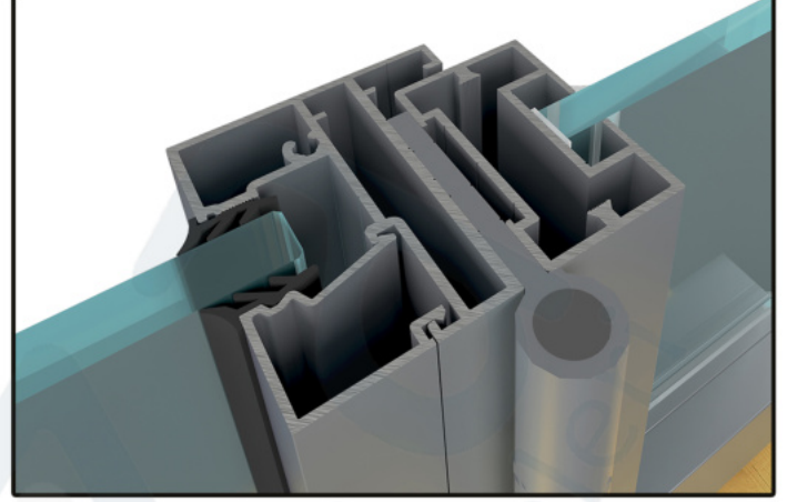
D20_SABİT CAMLI KAPI KASA + DÜZ CAM KANAT DETAYI
