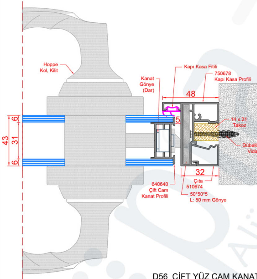
D56_ÇİFT YÜZ CAM KANAT + KAPI KASA DETAYI
