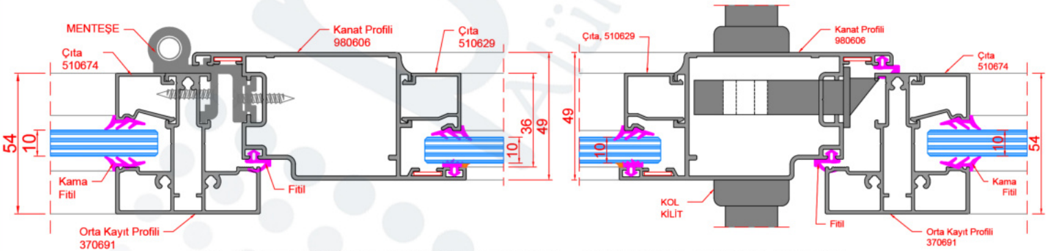
D44_SABİT CAMLI ORTA KAYIT PROFİLİNE + AÇILIR SİSTEM KANAT DETAYI
