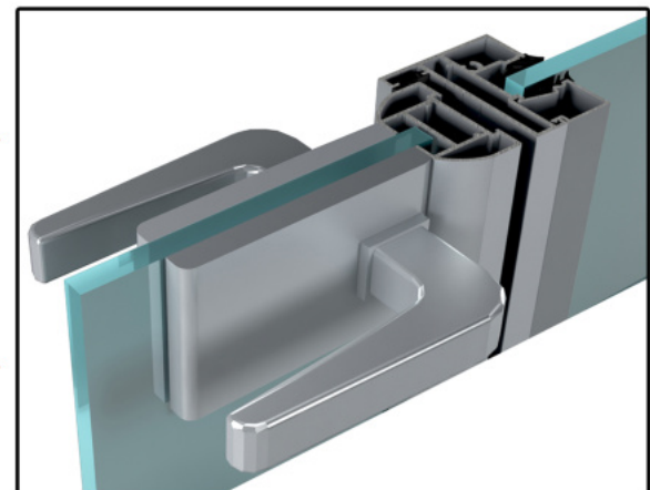
D50_OVAL CAM KANAT + SABİT CAMLI KAPI KASA DETAYI
