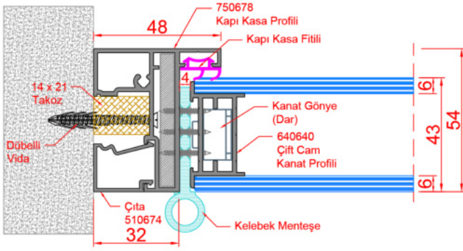
D55_KAPI KASA + ÇİFT YÜZ CAM KANAT DETAYI
