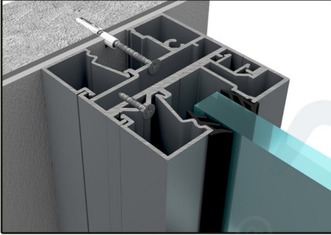
D40_DUVARA KAPI KASA PROFİLİ + KANAT ÜSTÜ SABİT CAM, ADAPTÖR PROFİL DETAYI
