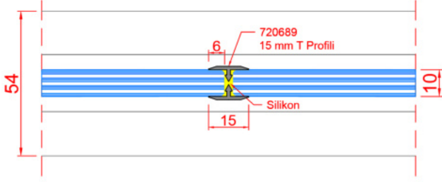
D65_15 MM T PROFİLİ İLE 10 MM CAM CAMA BİRLEŞİM DETAYI
