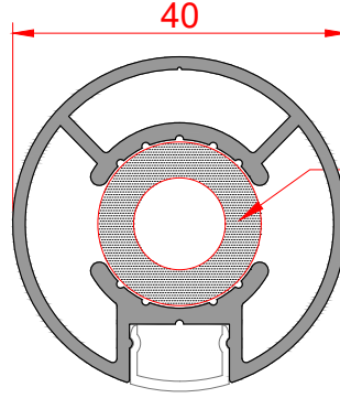
Profil No : 1006216 Ağırlık : 0,830 Kg/m
