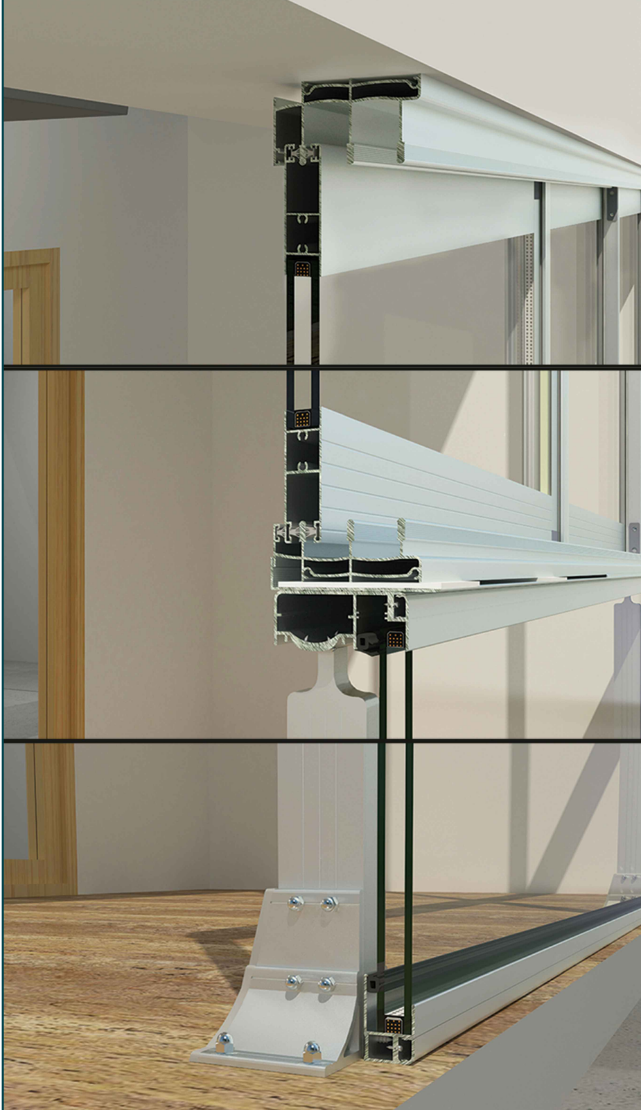
80*30 KÜPEŞTE, 90° KÖŞE
