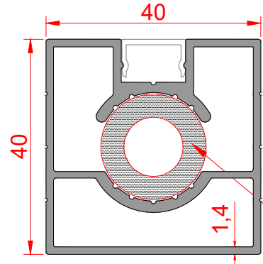
Profil No : 1006123 Ağırlık : 0,060 Kg/m
