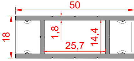
Profil No : 730667 Ağırlık : 0,630 Kg/m
