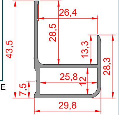
Profil No: 970691 Ağırlık: 0,520 Kg/m
