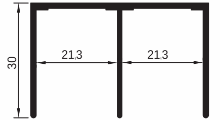
pr no:650646/86 0,500 kg/m
