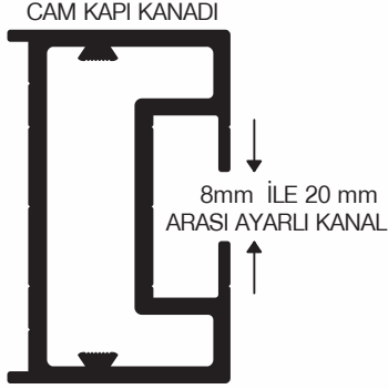
pr no:1006186/26 0.821 kg/m
