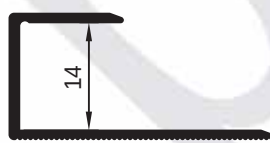
pr no:620667/109 0.195 kg/m
