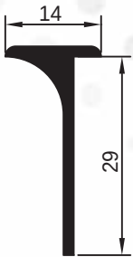
pr no:560609/104 0.215 kg/m
