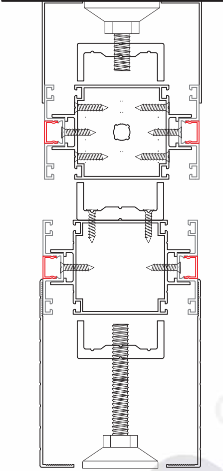
80 LİK SİSTEM DEMONTABLE ZEMİN VE TAVAN SIKIŞTIRMA DETAYI
