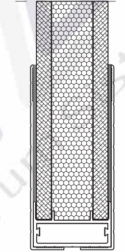
100 LÜK SİSTEM ALÜMİNYUM KASALI AHŞAP KAPI SÜPÜRGELİK DETAYI
