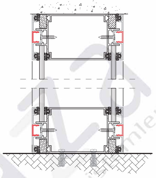
SÜPÜRGELİKSİZ 100 LÜK BÖLME TAVAN VE ZEMİN DETAYI
