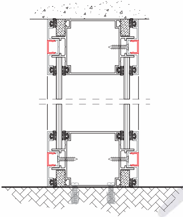
SÜPÜRGELİKSİZ 80 LİK BÖLME TAVAN VE ZEMİN DETAYI
