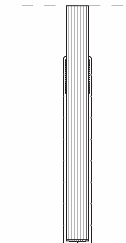
100 LÜK SİSTEM CAM KAPI SÜPÜRGELİK DETAYI
