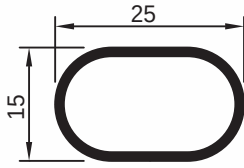
pr no:520631/98 0.200 kg/m
