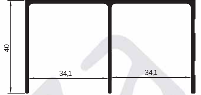
pr no:550627/86 0,685 kg/m
