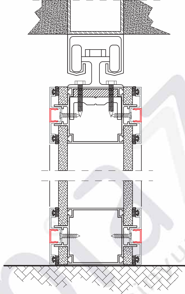
MEKAN BÖLÜCÜ KATLANIR PANEL SİSTEMİ ZEMİN VE TAVAN DETAYI
