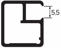
pr no:680612/94 0,285 gr/m
