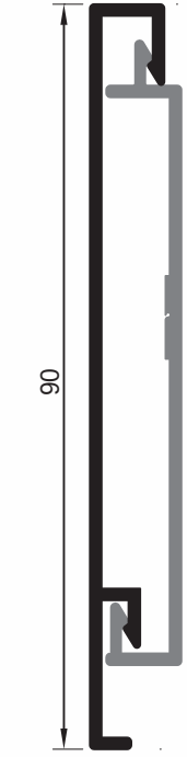
pr no:520696/81 0.455 kg/m
