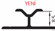
pr no:1006206/5 0.170 gr/m
