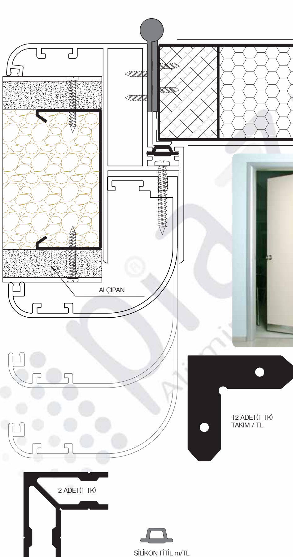
TEKMELİK DETAYI 1/2
