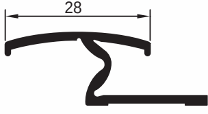
pr no:160605/109 0.275 kg/m
