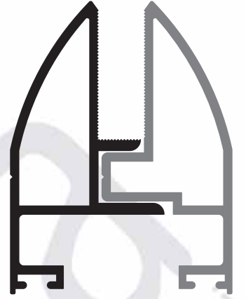
pr no:510663/68 0.589 kg/m
