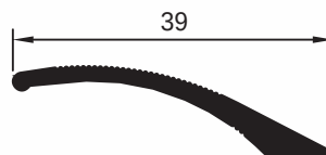
pr no:370634/108 0.245 kg/m
