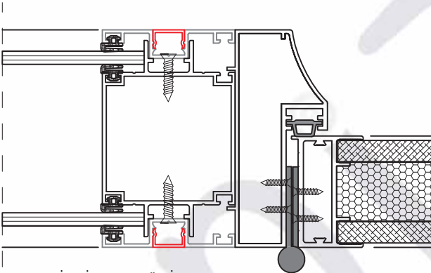
80 LİK SİSTEM ALÜMİNYUM KASALI AHŞAP KAPI DETAYI
