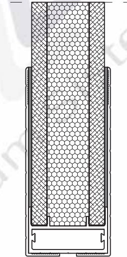
80 LİK SİSTEM ALÜMİNYUM KASALI AHŞAP KAPI SÜPÜRGELİK DETAYI
