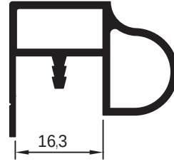
pr no:630665/88 0,395 kg/m
