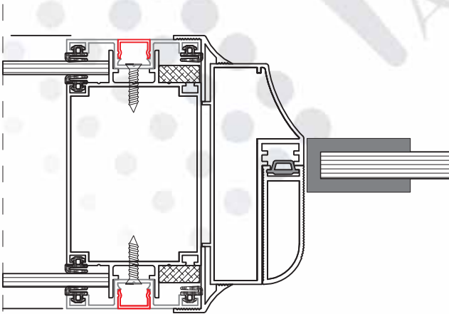
100 LÜK SİSTEMDE POMPALI KAPI KASASI DETAYI
