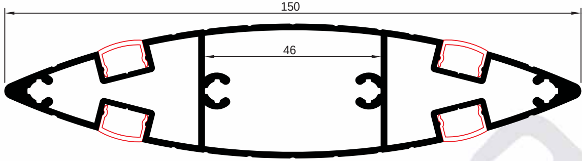
YENİ DEKORLU PLAZMA AYAĞI
