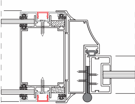
100 LÜK SİSTEM ALÜMİNYUM KASALI CAM KAPI DETAYI
