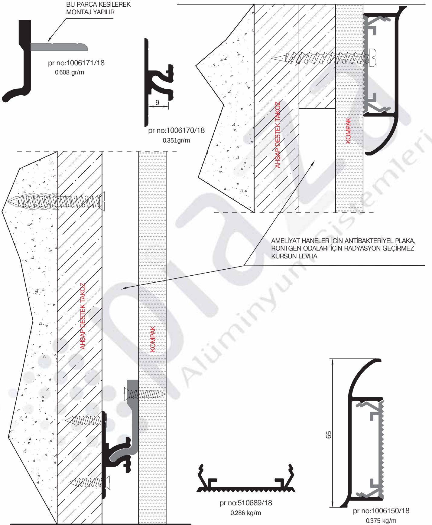
ZEMİN DETAY
