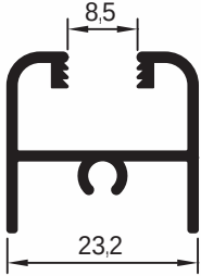
pr no:550629/86 0,280 kg/m
