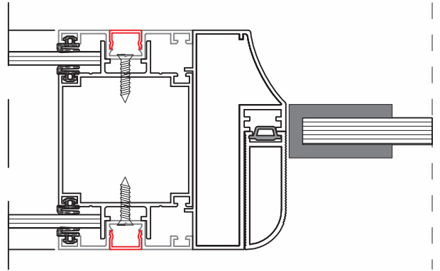
80 LİK SİSTEMDE POMPALI KAPI KASASI DETAYI
