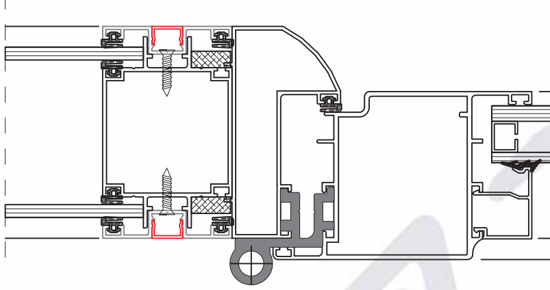
80 LİK SİSTEMDE ALÜMİNYUM KAPI DETAYI
