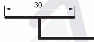
pr no:290638/109 0.165 kg/m
