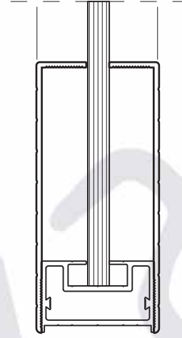
80 LİK SİSTEM ALÜMİNYUM KASALI CAM KAPI SÜPÜRGELİK DETAYI
