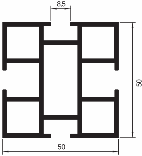
pr no:690632/58 1.650 gr/m
