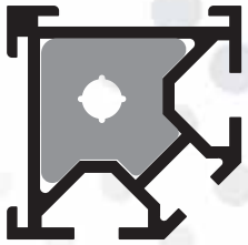
pr no:510660/58 0.478 gr/m
