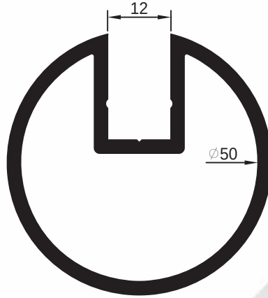
pr no:1106098/70 1.266 kg/m
