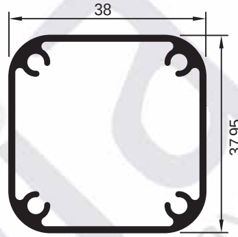
pr no:630652/77 0.560 kg/m
