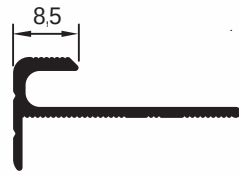
pr no:370628/109 0.165 kg/m
