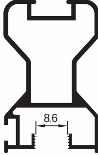
pr no:520632/86 0,610 kg/m
