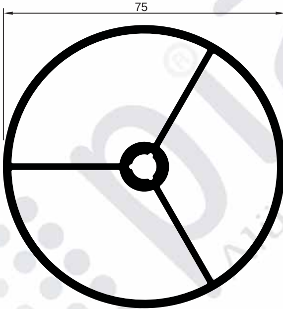
pr no:510681/75 1.844 kg/m
