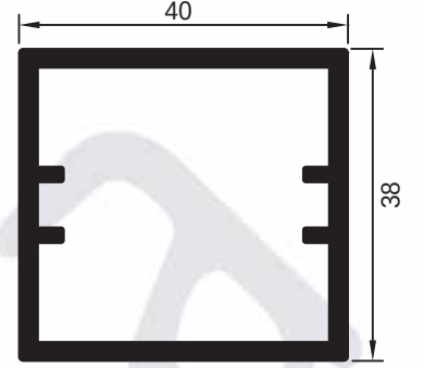
pr no:380632/77 0.975 kg/m
