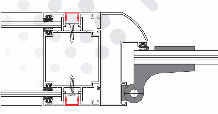
80 LİK SİSTEM CAM KAPI DETAYI
