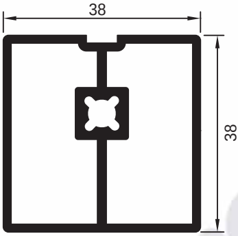
pr no:380642/77 0.840 kg/m
