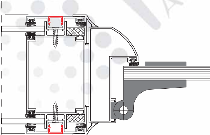
100 LÜK SİSTEM CAM KAPI DETAYI
