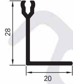
pr no:800659/119 0,222 gr/m
