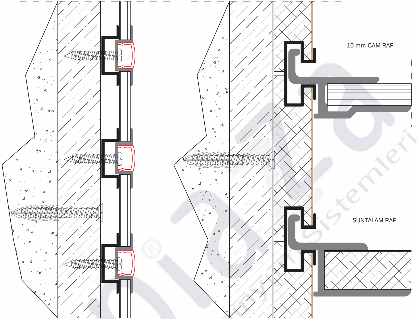
DUVAR VE TAVANA AYNALI ve CAMLİ LAMBİRİ UYGULAMA DETAYI
