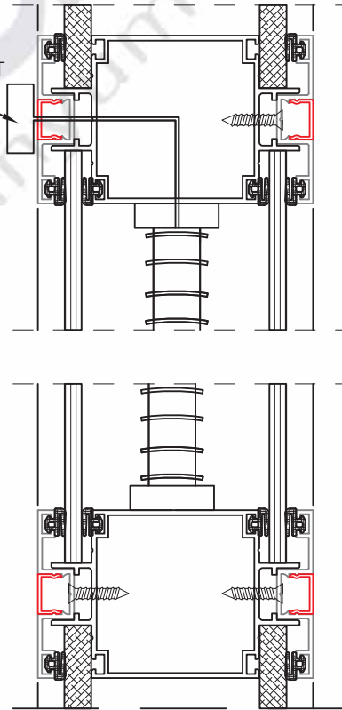
80 LİK SİSTEM DEKORSUZ JALUZİ DETAYI
