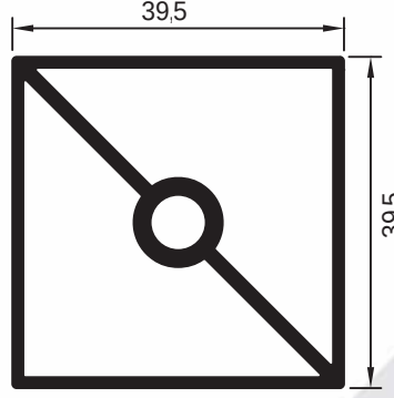
pr no:690617/77 0.860 kg/m
