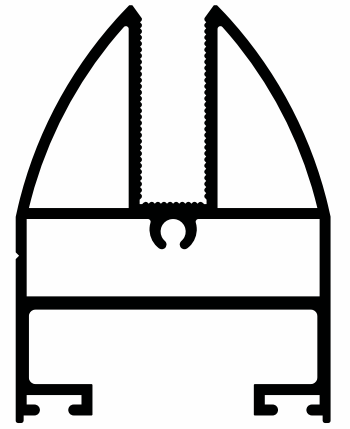
pr no:510673/68 1.566 kg/m
