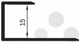
pr no:620628/109 0.200 kg/m
