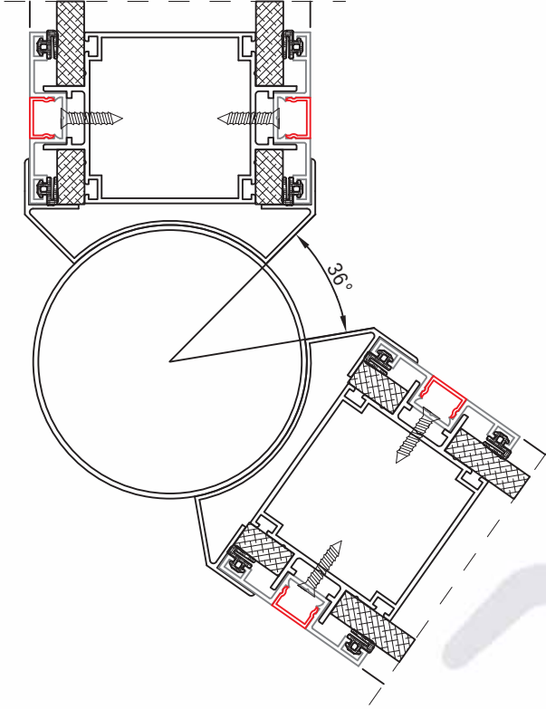
80 LİK SİSTEM ÇOK AÇILI KÖŞE DÖNÜŞ
