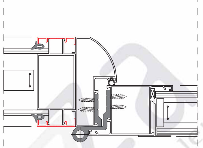
İki CAM ARASI JALUZİ KESİT DETAYI
