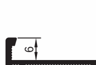
pr no:370639/109 0.097 kg/m
