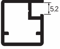
pr no:570605/94 0,290 kg/m
