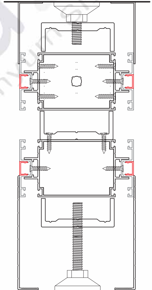
100 LÜK SİSTEM DEMONTABLE ZEMİN ve TAVAN SIKIŞTIRMA DETAYI
