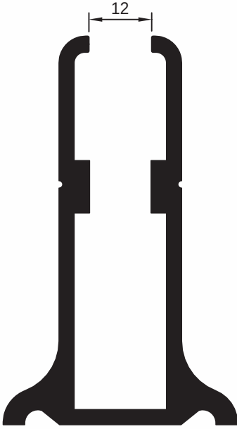
pr no:800675/70 1.752 kg/m
