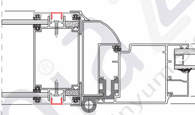
100 LÜK SİSTEMDE ALÜMİNYUM KAPI DETAYI
