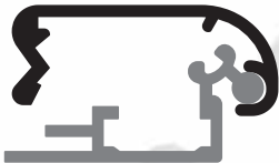
pr no:550675/113 0.216 kg/m
