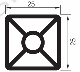
pr no:370606/77 0.650 kg/m
