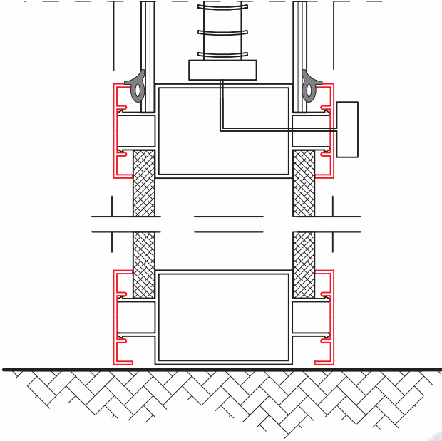
İki CAM ARASI JALUZİ ZEMİN DETAYI
