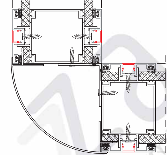
80 LİK SİSTEM 90 DERECE KÖŞE DÖNÜŞ DETAYI
