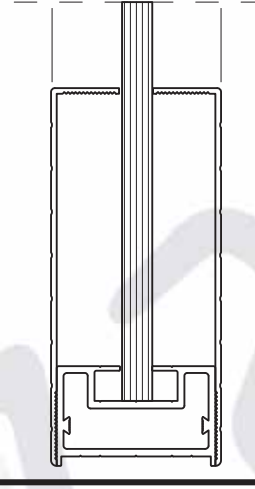
100 LÜK SİSTEM ALÜMİNYUM KASALI CAM KAPI SÜPÜRGELİK DETAYI
