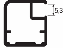
pr no:570628/94 0,295 kg/m
