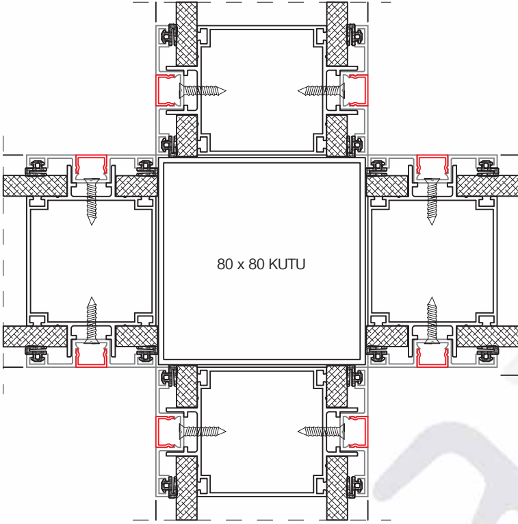
80 LİK SİSTEM DÖRT KÖŞE KESİT DETAYI
