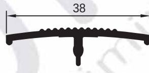
pr no:170603/108 0.205 kg/m
