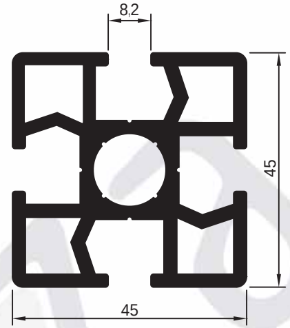
pr no:170625/58 2.055 gr/m
