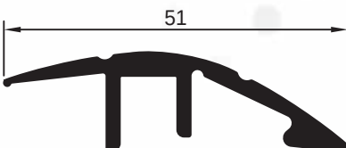
pr no:680610/108 0.475 kg/m
