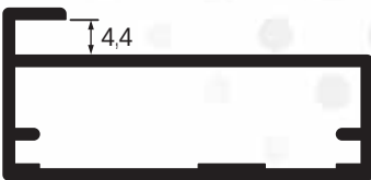
pr no:440637/94 0,490 kg/m
