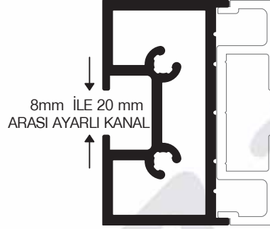
pr no:1006175/26 0.845 kg/m
