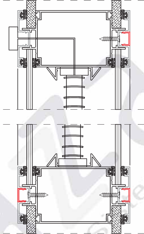
100 LÜK SİSTEM DEKORLU JALUZİ DETAYI
