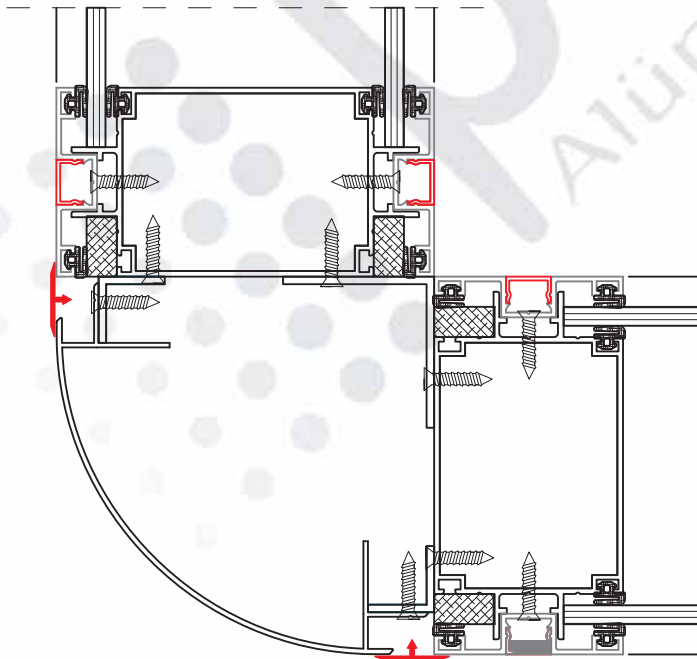
100 LÜK SİSTEM 90 DERECE KÖŞE DÖNÜŞ DETAYI
