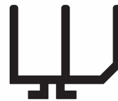
pr no:500663/58 0.267 gr/m
