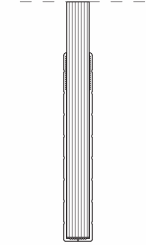
80 LİK SİSTEM CAM KAPI SÜPÜRGELİK DETAYI
