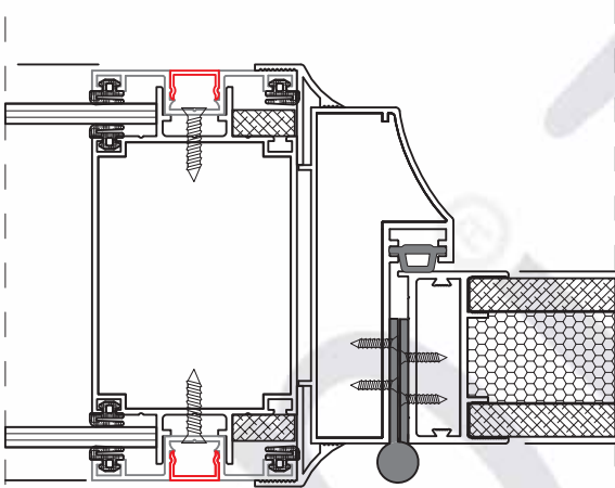
100 LÜK SİSTEM ALÜMİNYUM KASALI AHŞAP KAPI DETAYI
