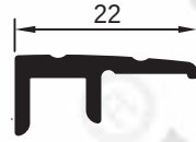
pr no:680606/109 0.170 kg/m
