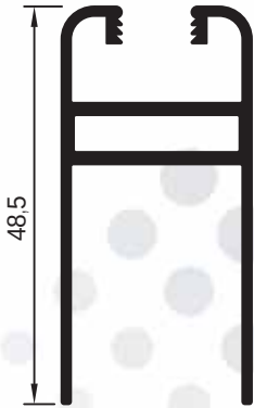
pr no:550631/86 0,535 kg/m
