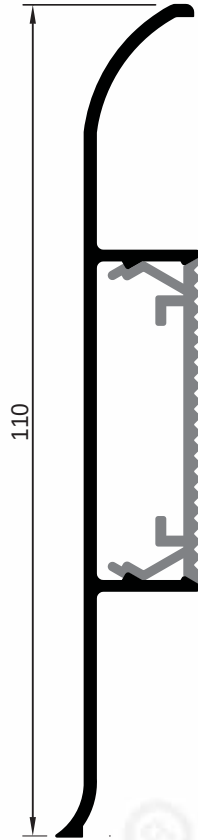
pr no:510685/80 0.583 kg/m
