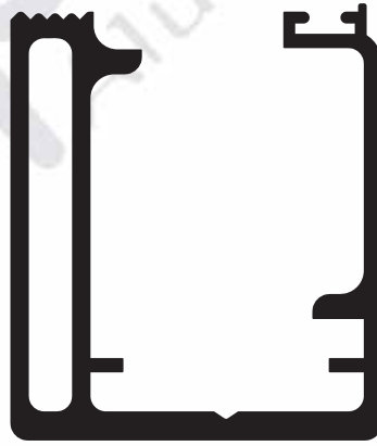
pr no:510668/68 1.426 kg/m
