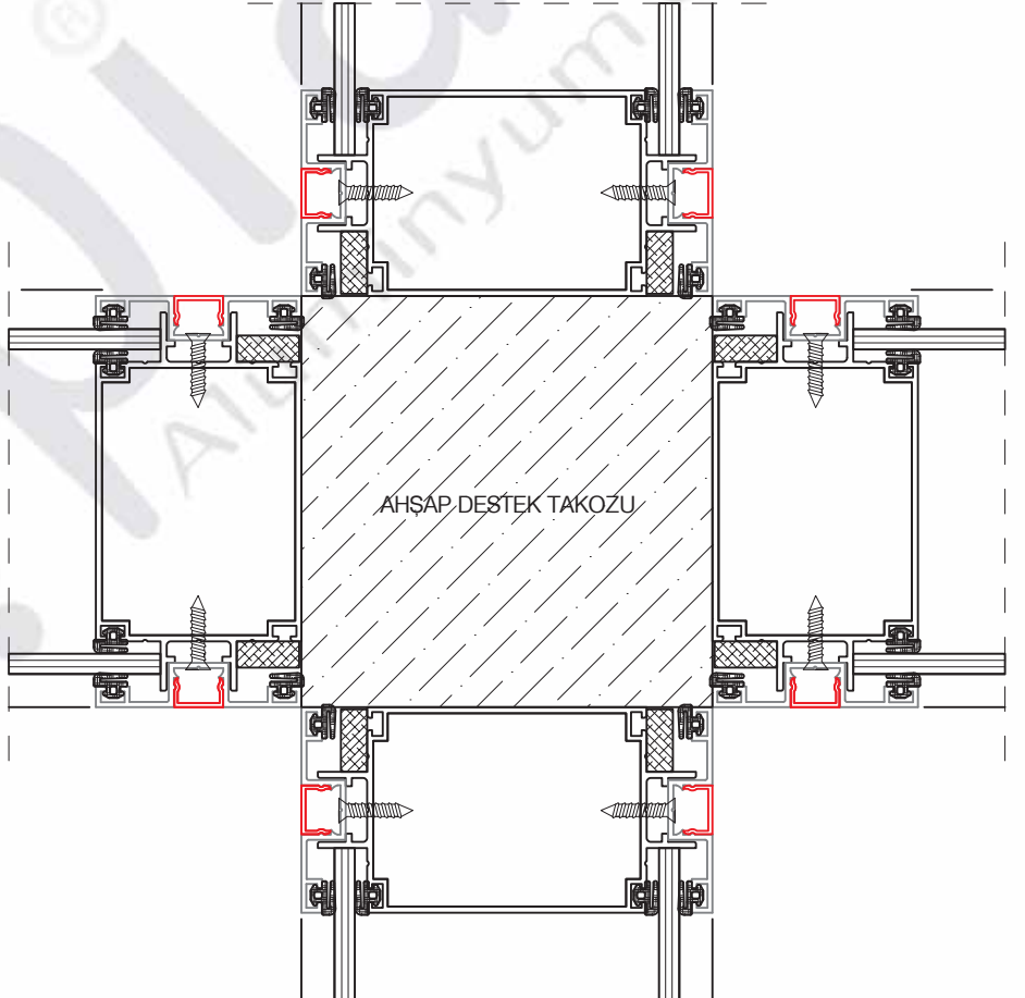
100 LÜK SİSTEM DÖRT KÖŞE KESİT DETAYI
