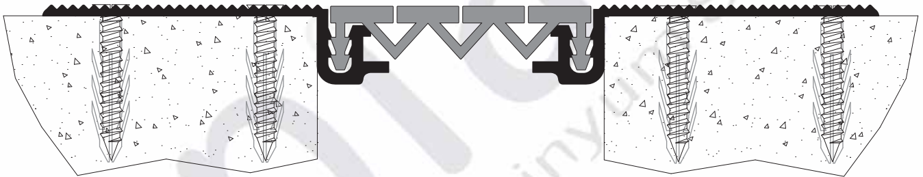
İKİ ZEMİN ARASI DİLATASYON DETAYI
