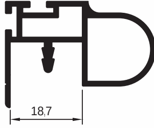
pr no:630662/88 0,545 kg/m
