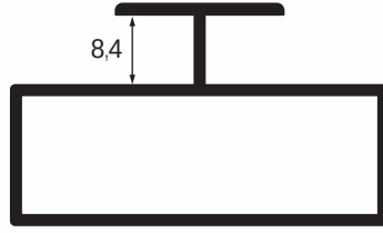
pr no:430641/95 0,416 kg/m
