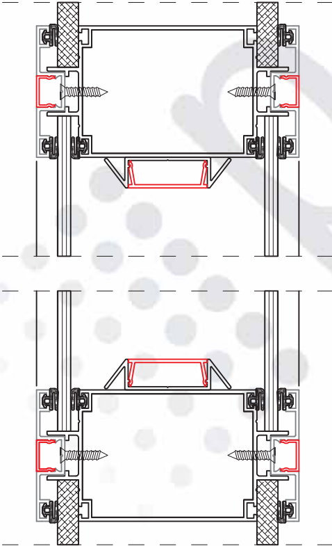
100 LÜK SİSTEM DEKORLU DETAYI
