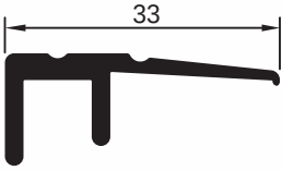
pr no:680609/109 0.275 kg/m
