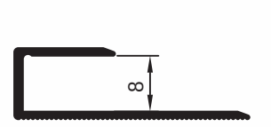
pr no:620626/109 0.175 kg/m
