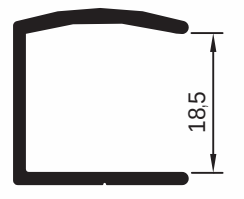
pr no:560653/88 0,270 kg/m
