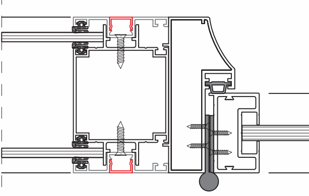
80 LİK SİSTEM ALÜMİNYUM KASALI CAM KAPI DETAYI
