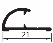
pr no:630670 0,115 kg/m
