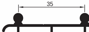
pr no:550655/86 0,310 kg/m
