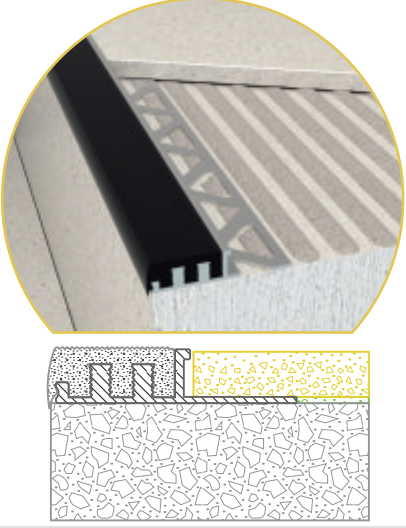
3806492 - Basamak profili
