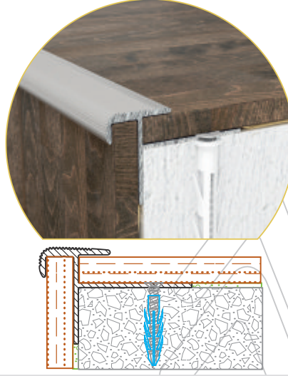
290635 - Basamak profili
